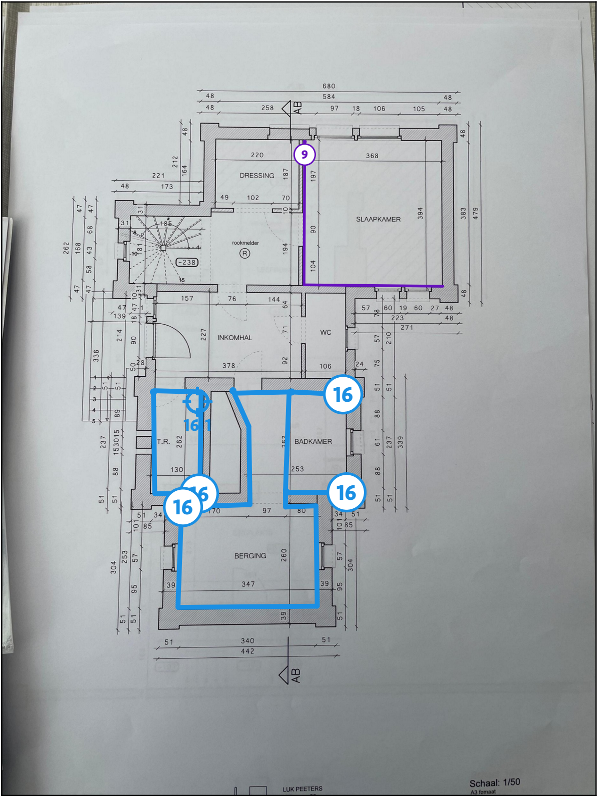
Legende van plan 1.5: Grondplan sous sol Muren
