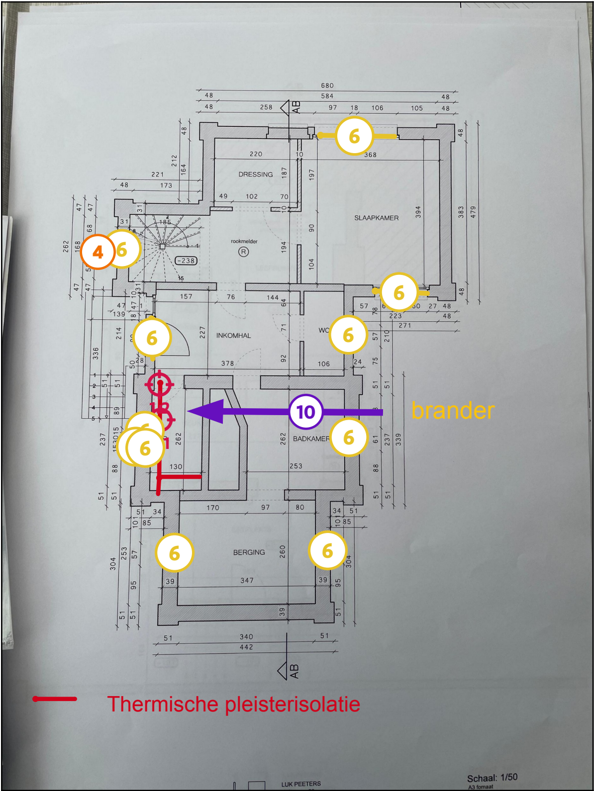
Legende van plan 1.2: Grondplan sous sol
