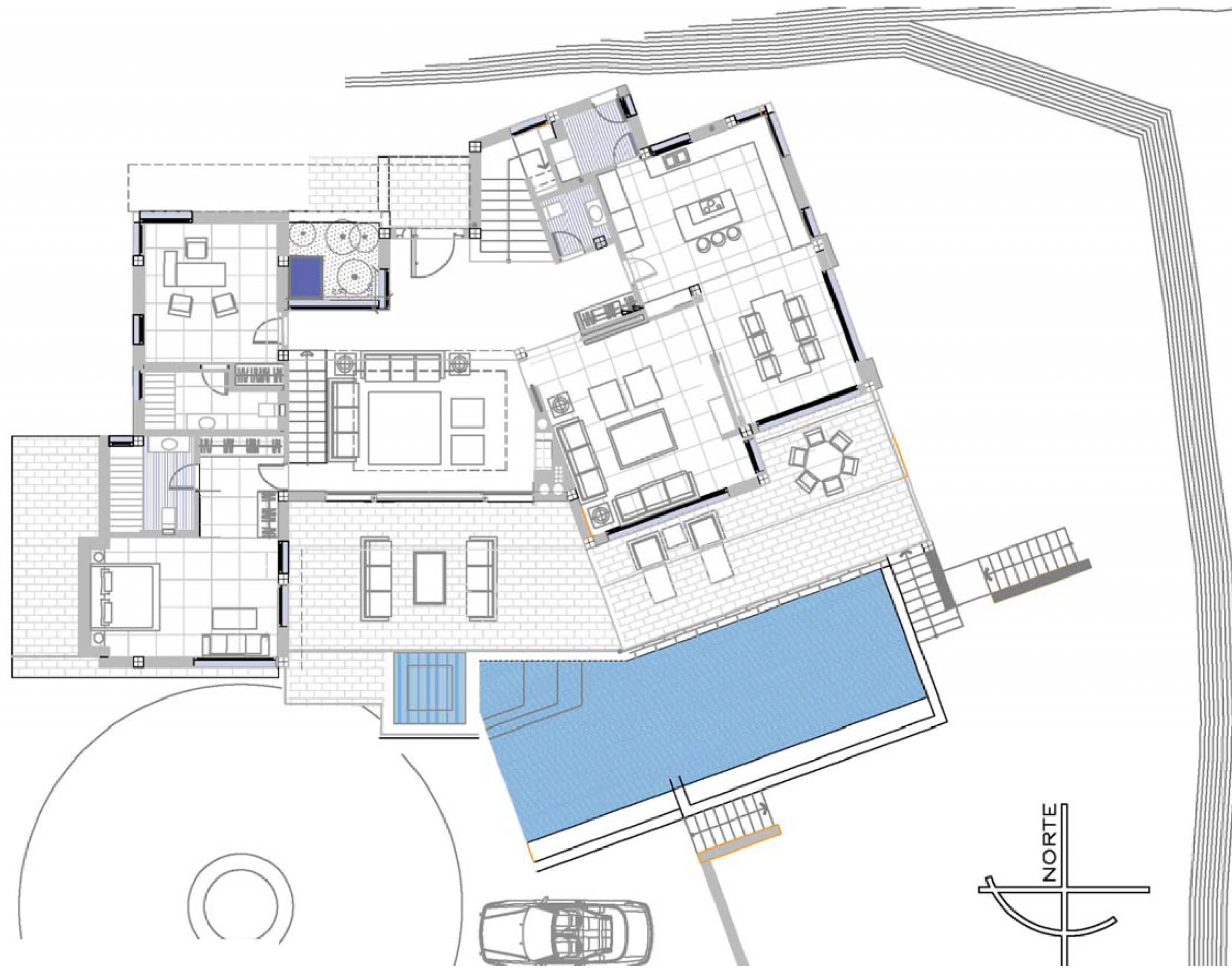
PLANTA BAJA
