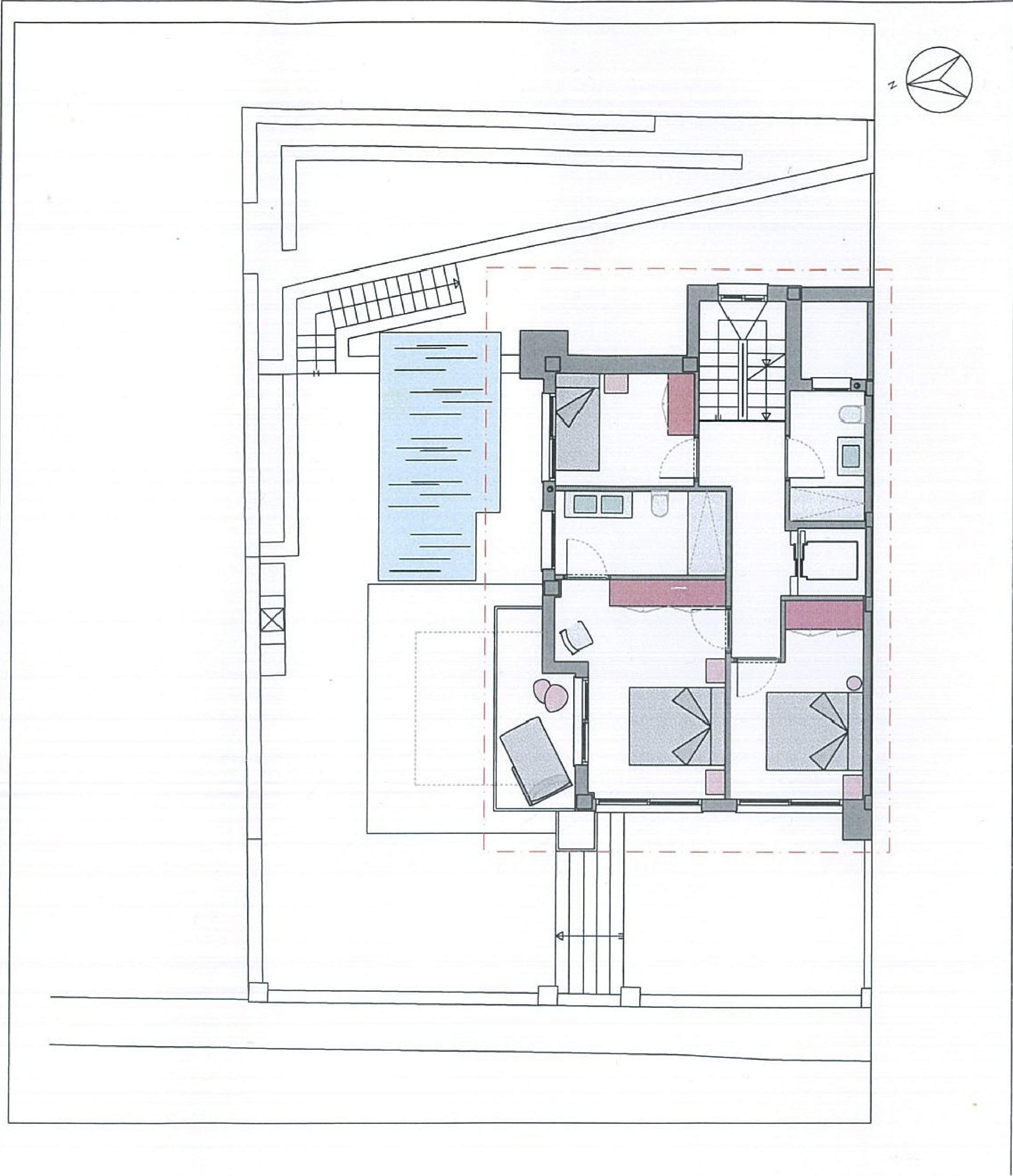
PLANTA DE DISTRIBUCIÓN Y SUPERFICIES.
