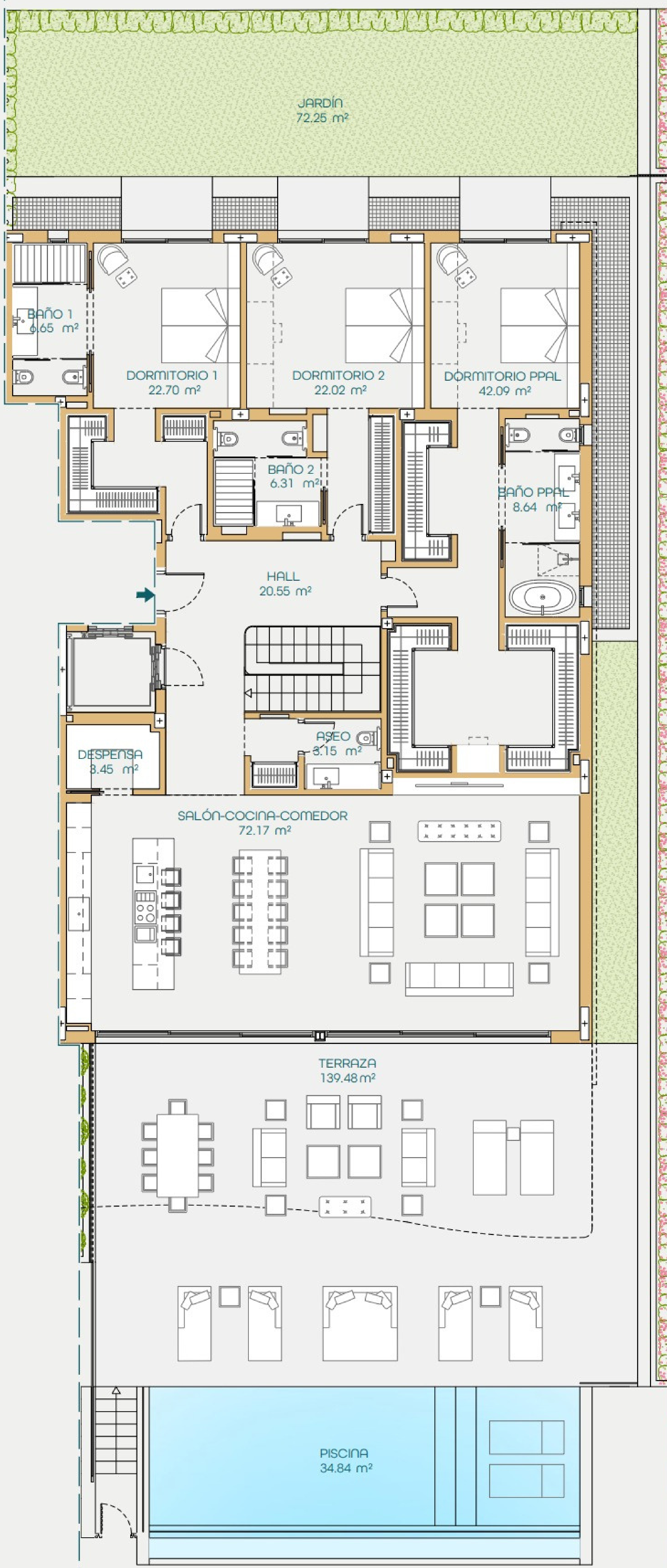
PLANTA BAJA
