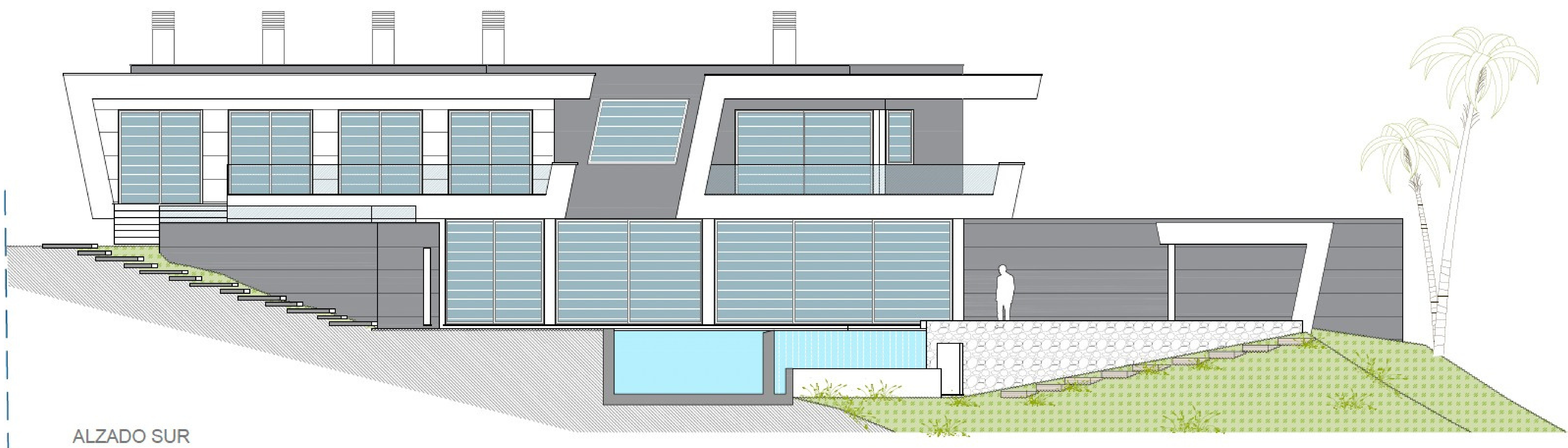
ALZADO SUR
