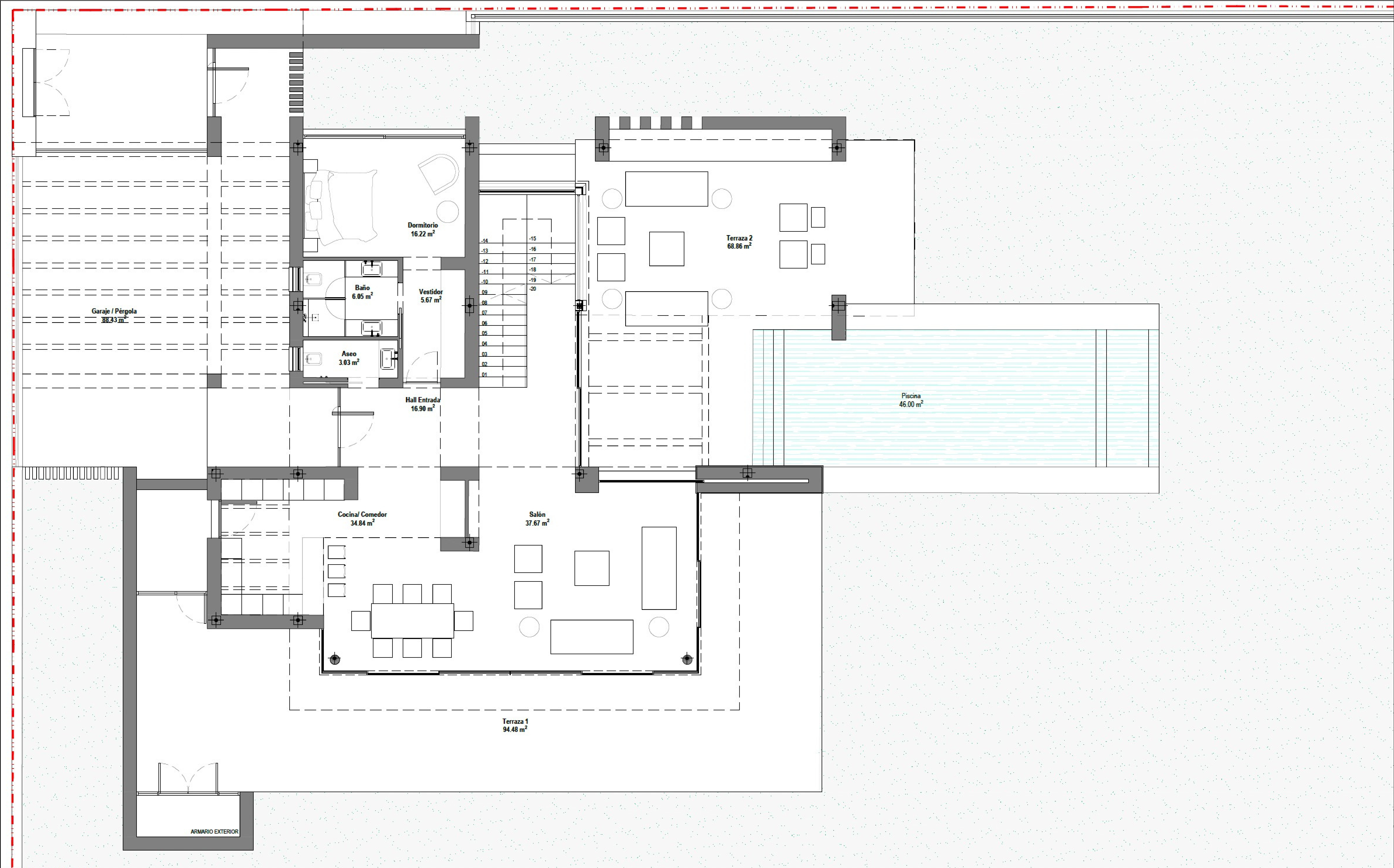
PLANTA BAJA_E:1.50
