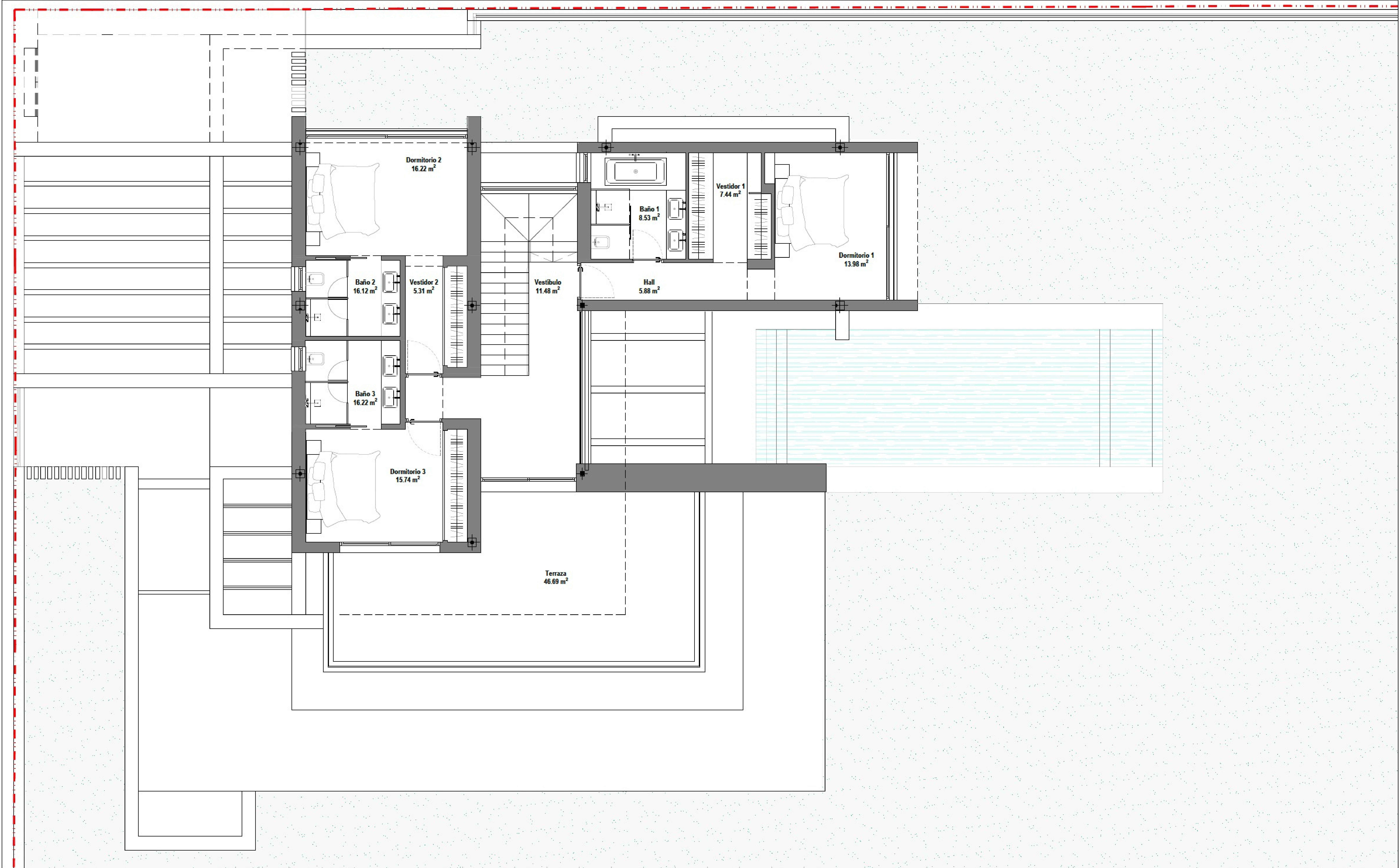
PLANTA PRIMERA_E:1.50
