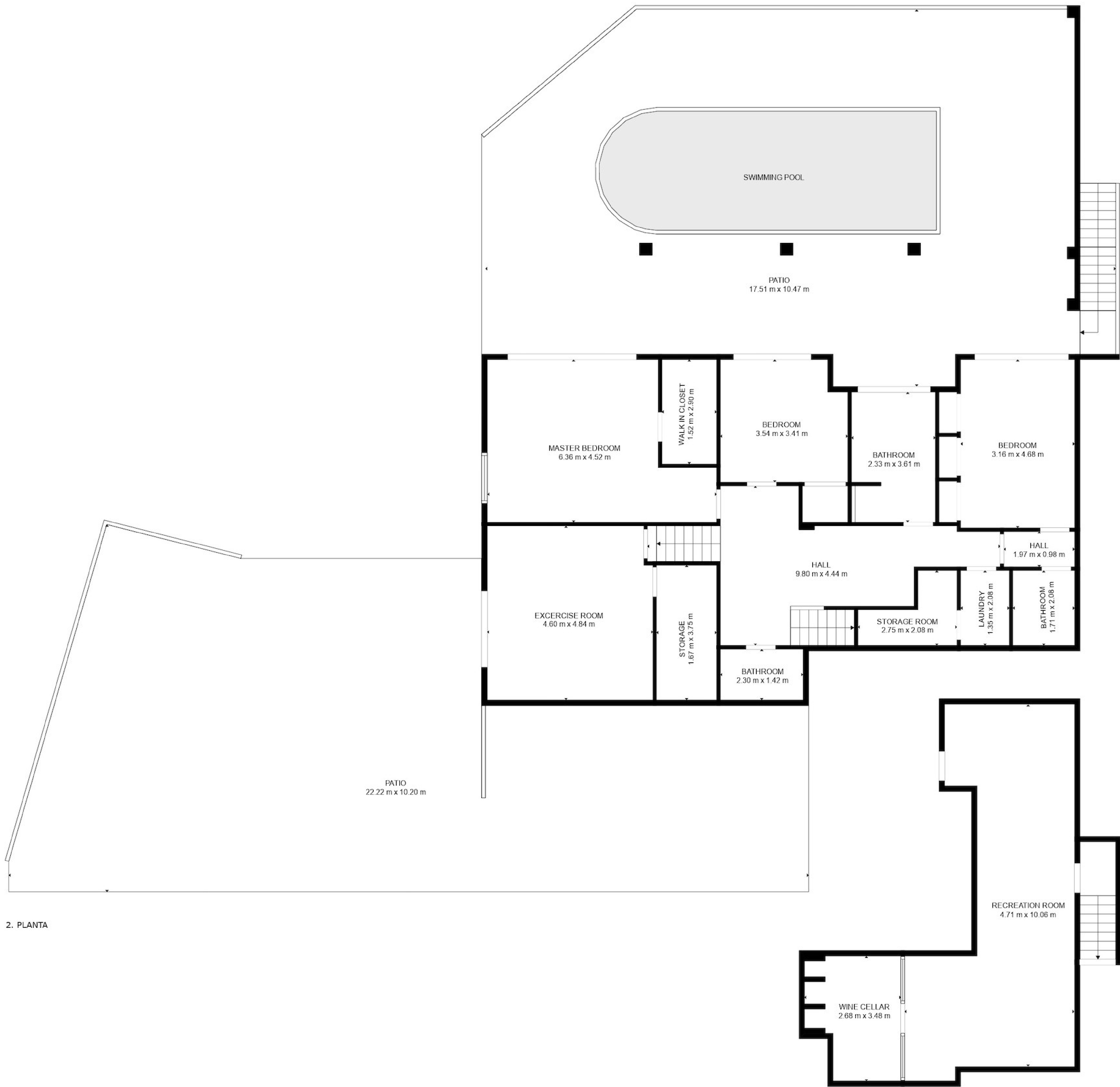
1. PLANTA
