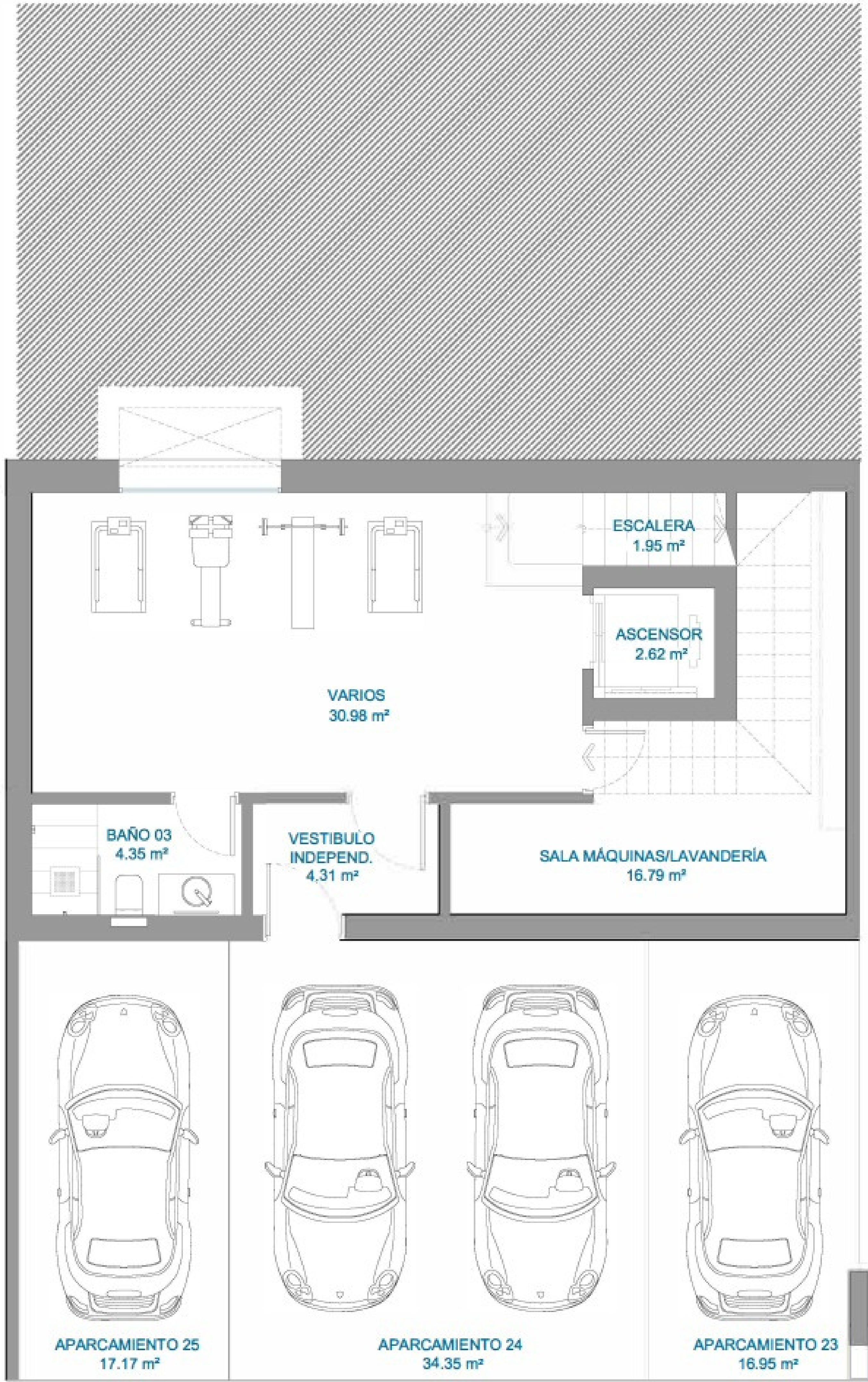
PLANTA SOTANO
