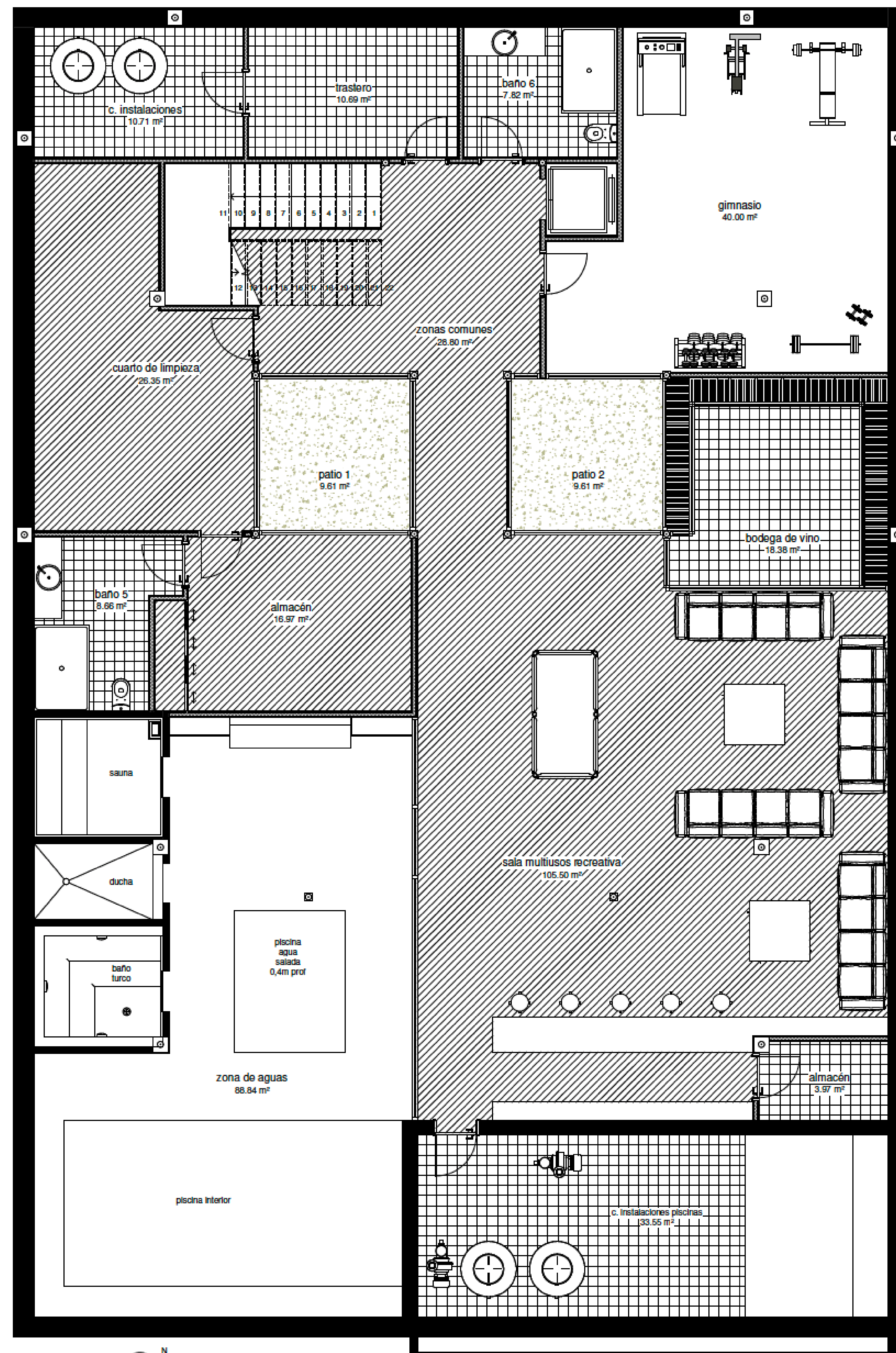
- PLANTA SÓTANO
