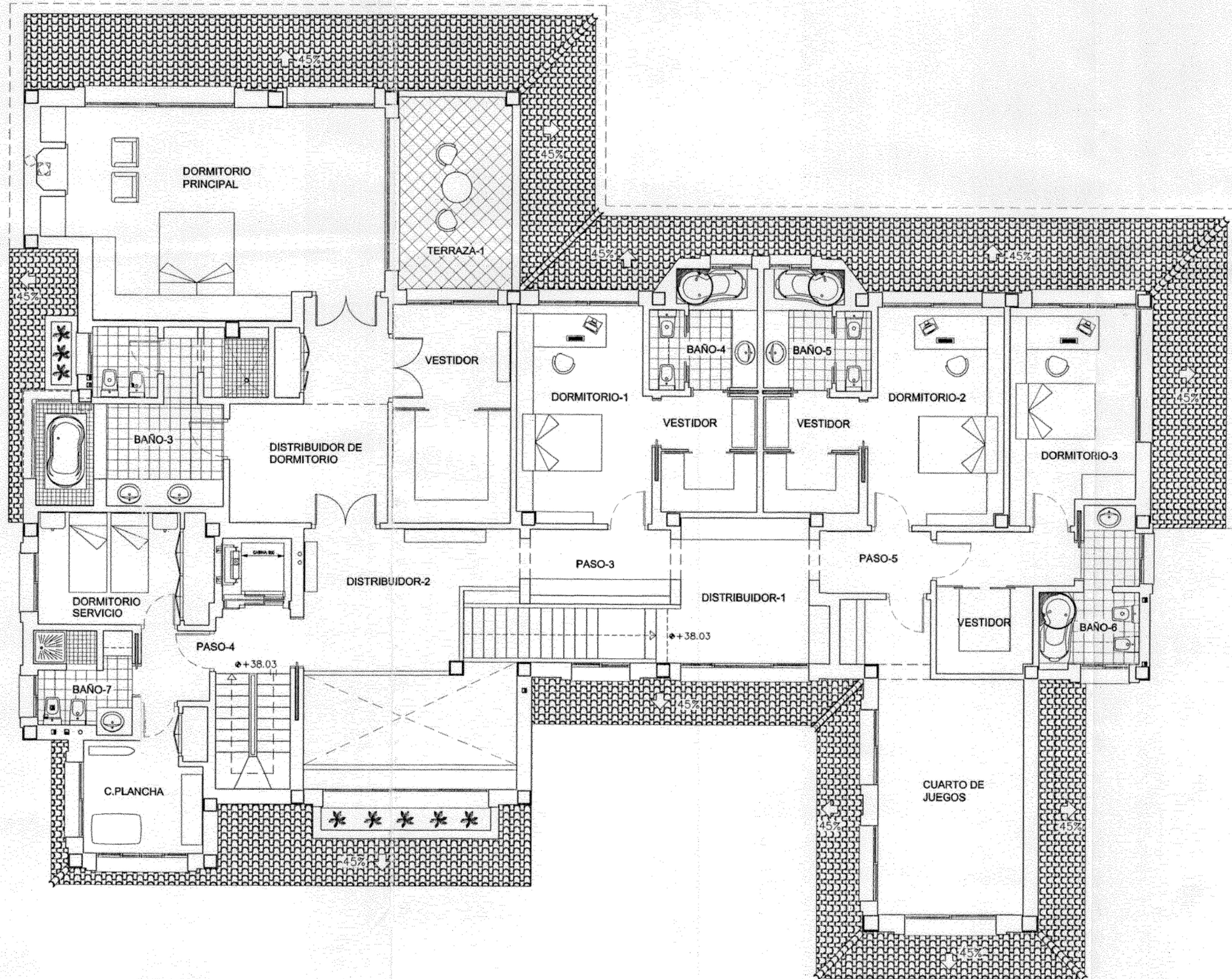
PLANTA PRIMERA
