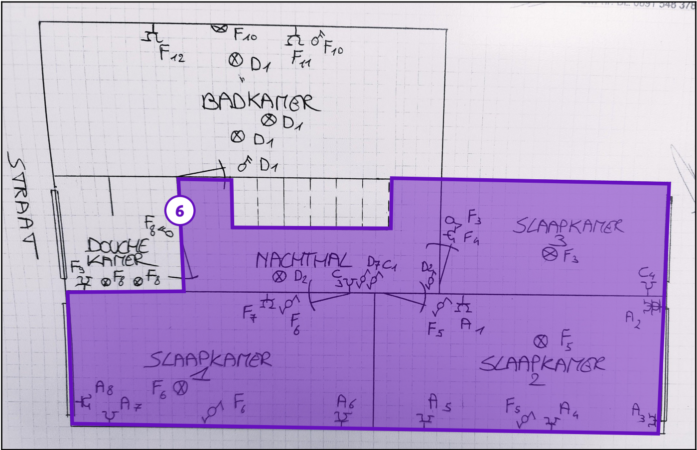
Legende van plan 1.8: vloerplan v+1
