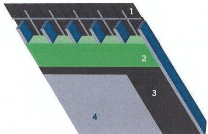
1. Onderdak | 2. Isolatie | 3. Dampscherm | 4. binnenafwerking
