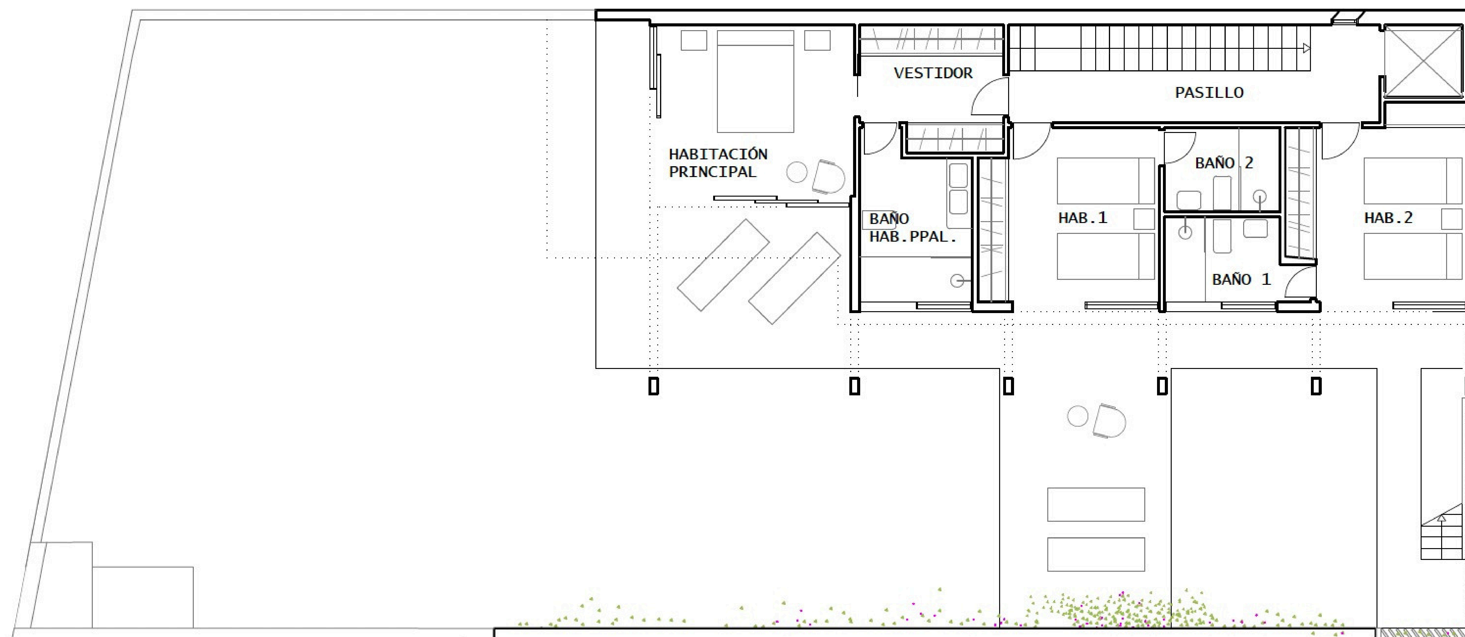
PLANTA PRIMERA E:1/150
