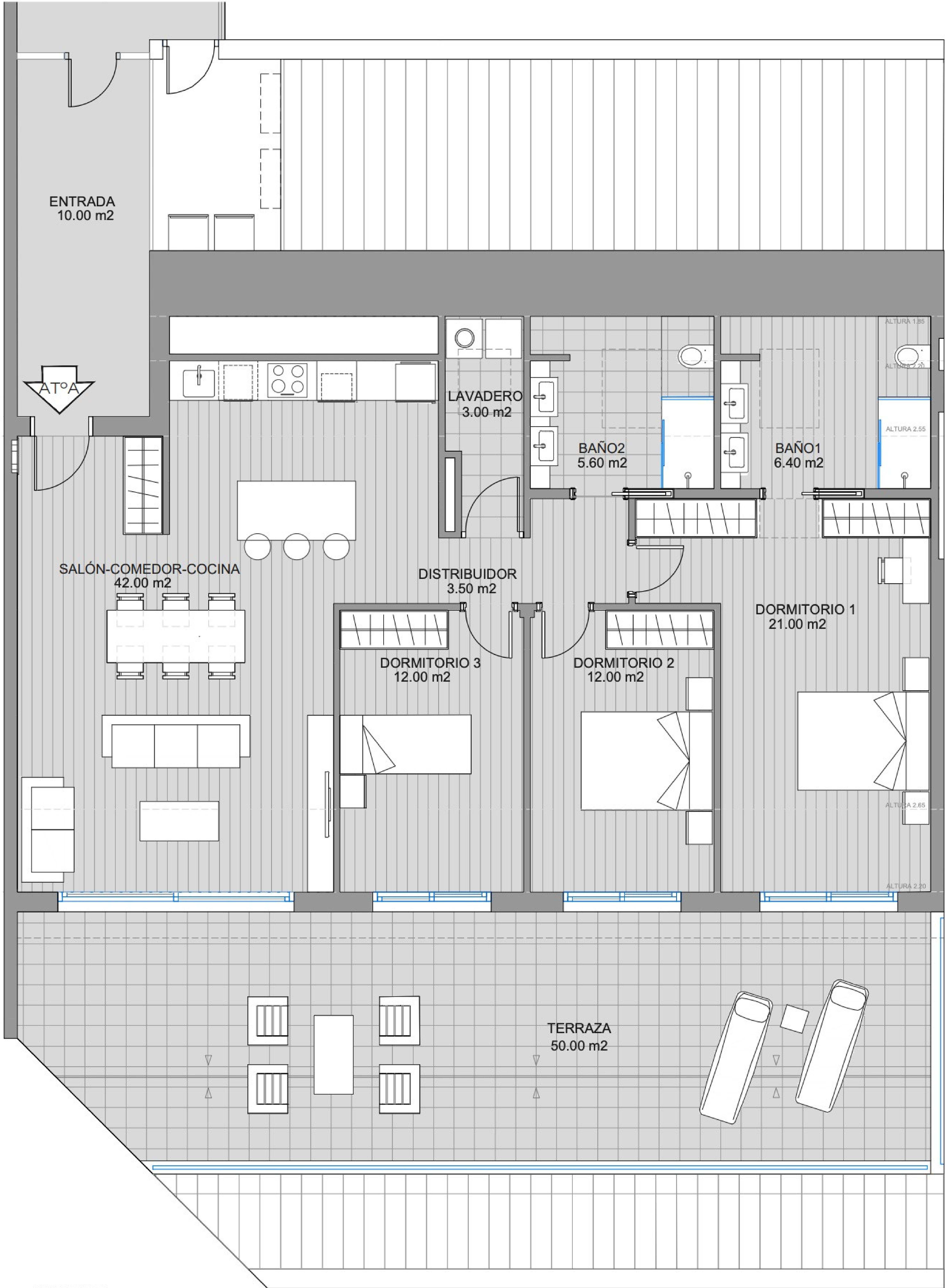
VIVIENDA E: 1/75
