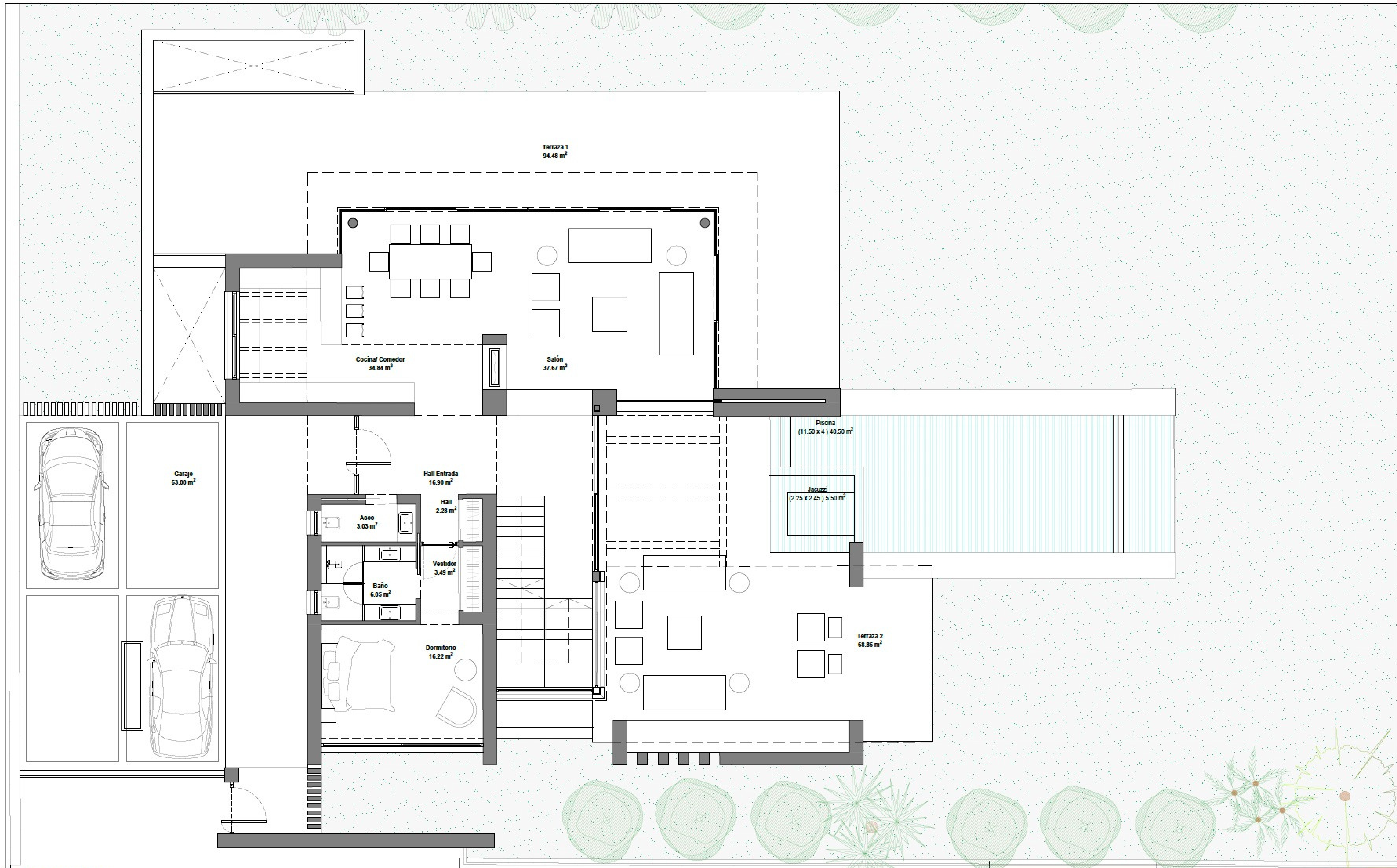
PLANTA BAJA_E:1.50
