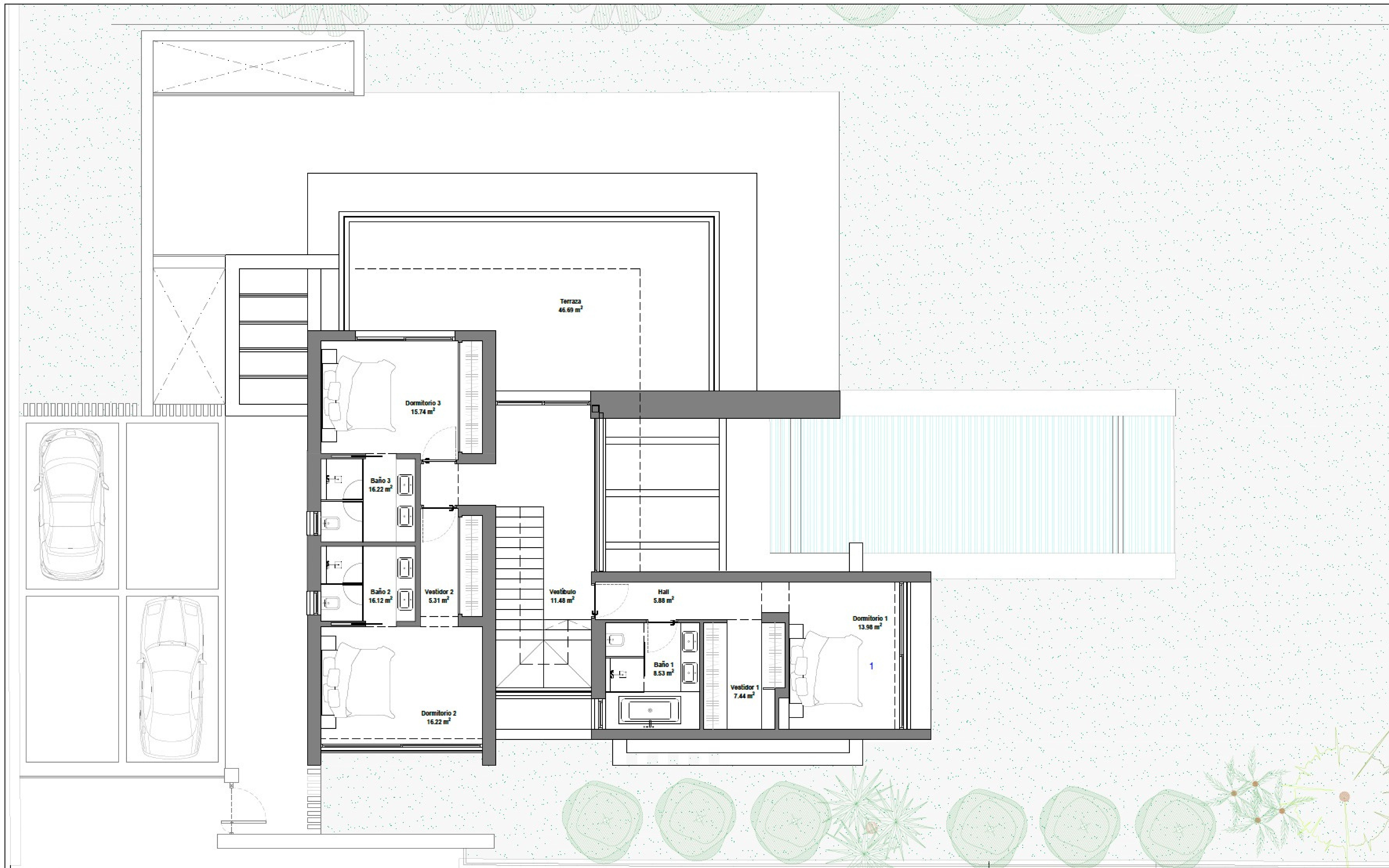
PLANTA PRIMERA_E:1.50
