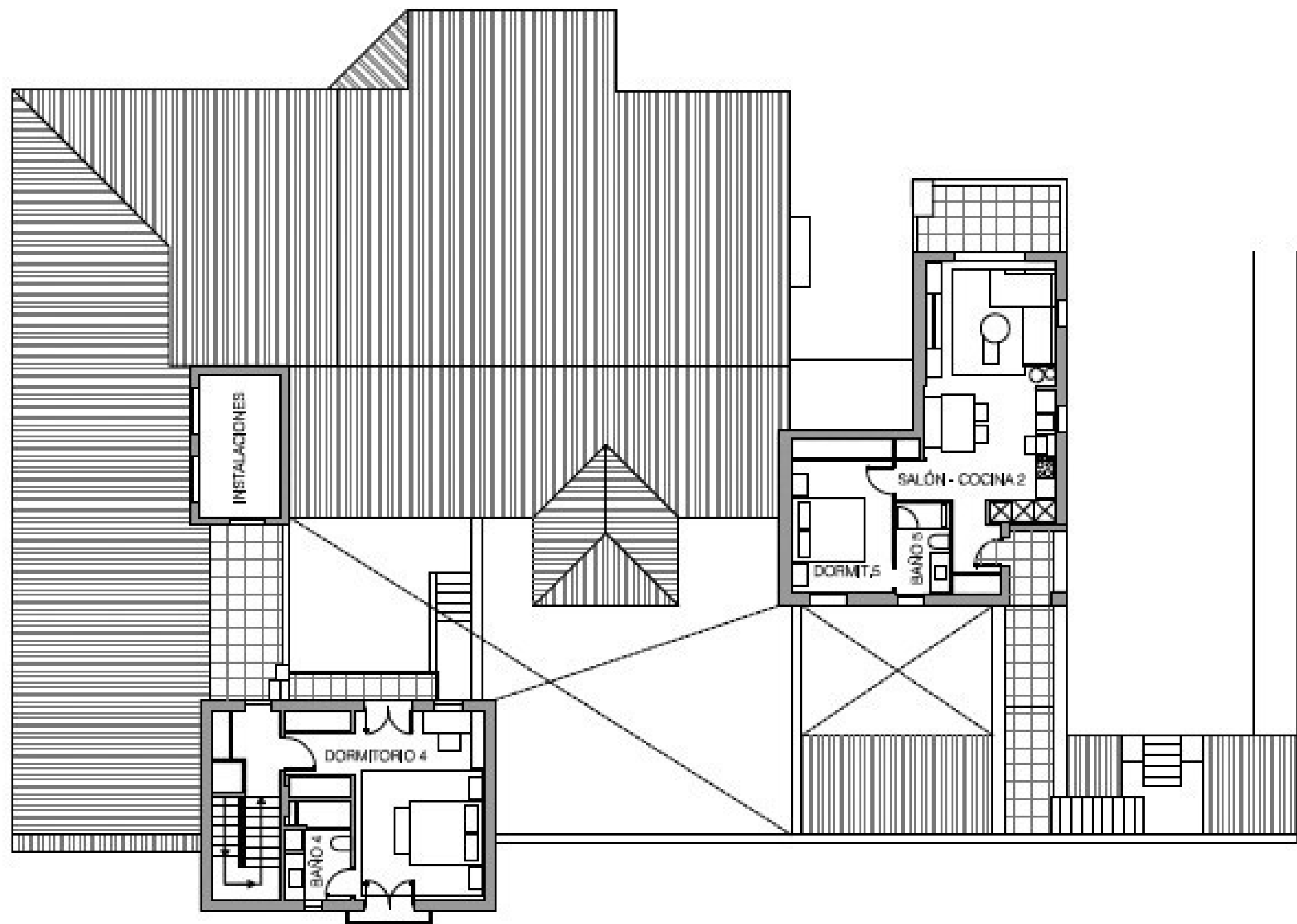
PLANTA ALTA
