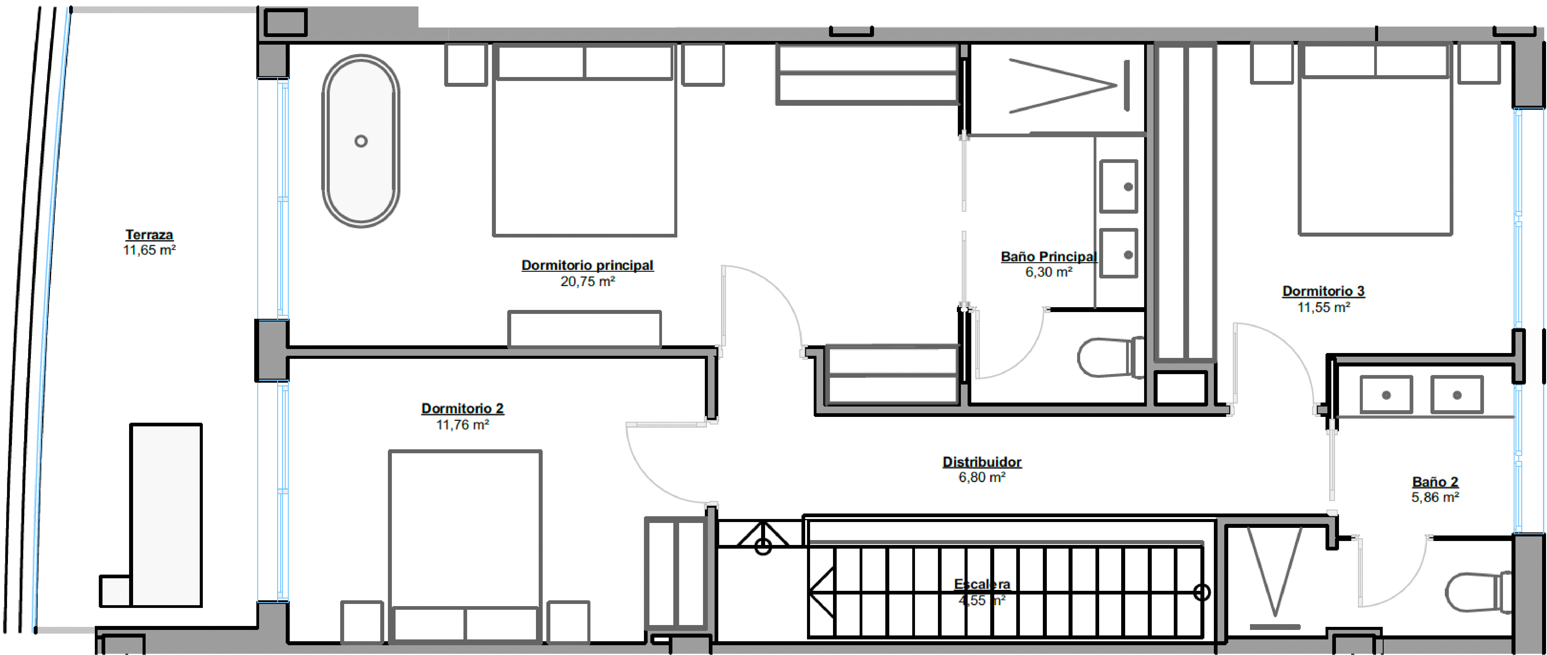
PLANTA PRIMERA
