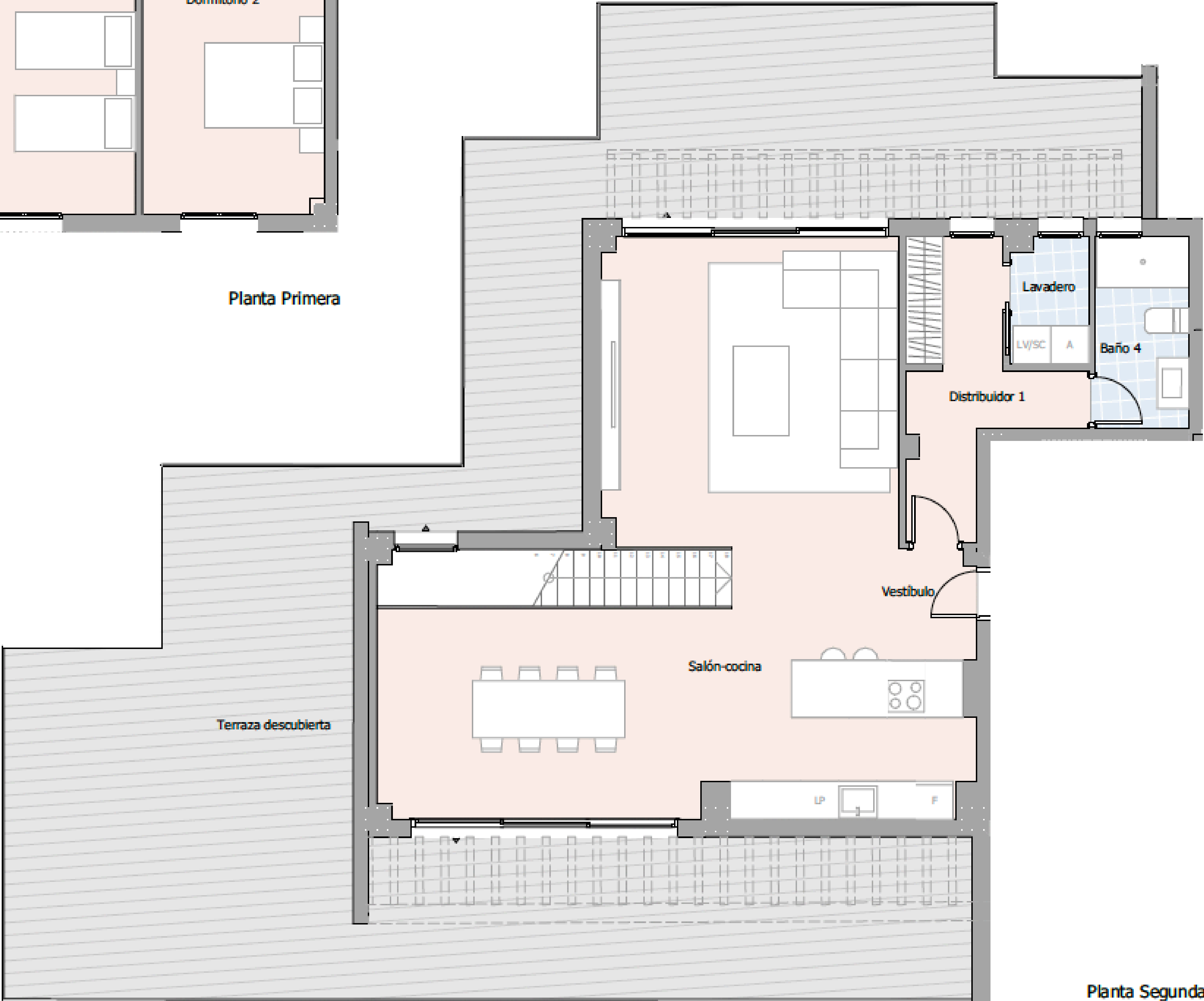
Planta Segunda
