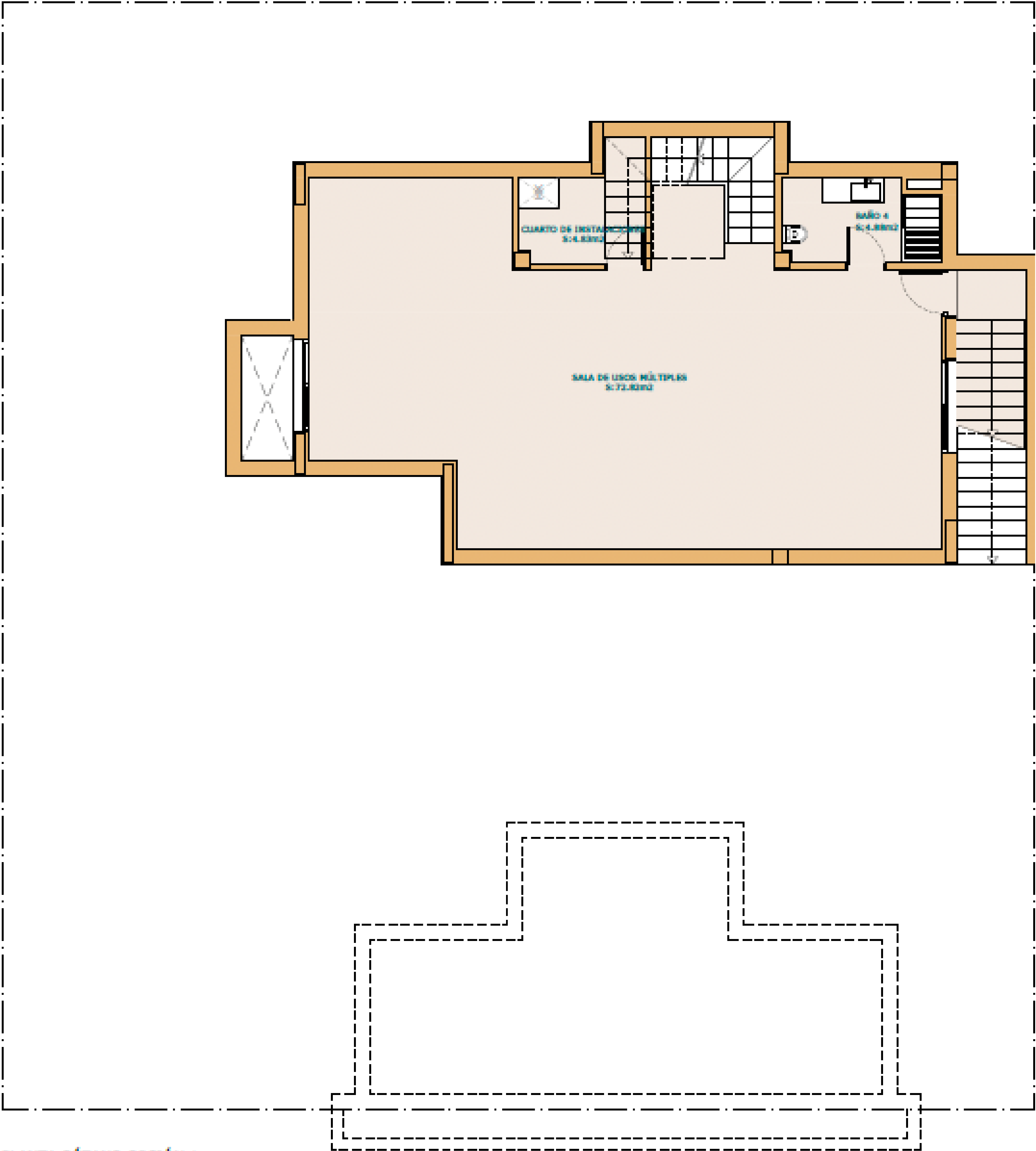
PLANTA SÓTANO OPCIÓN 1
