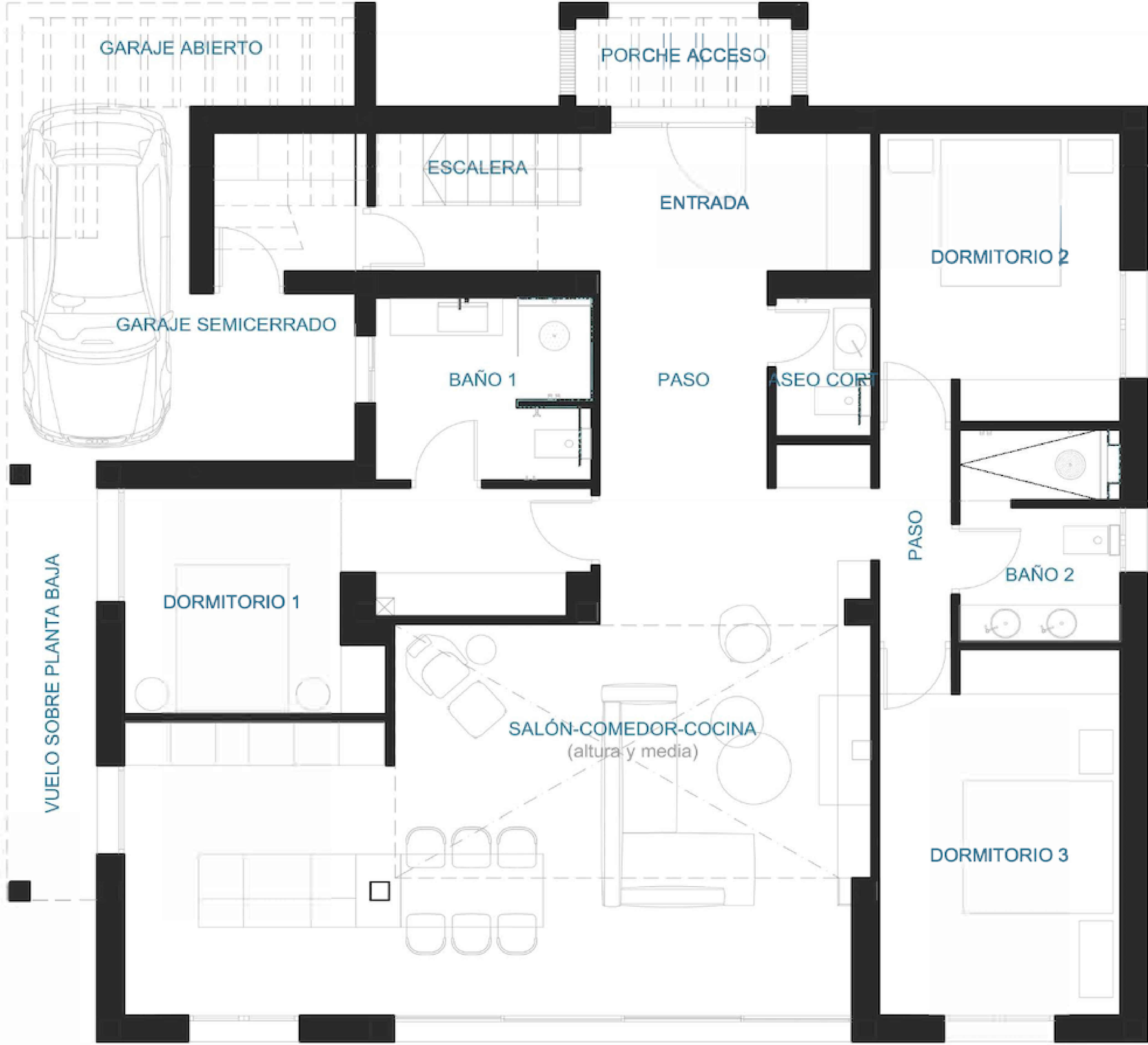
PLANTA BAJA
