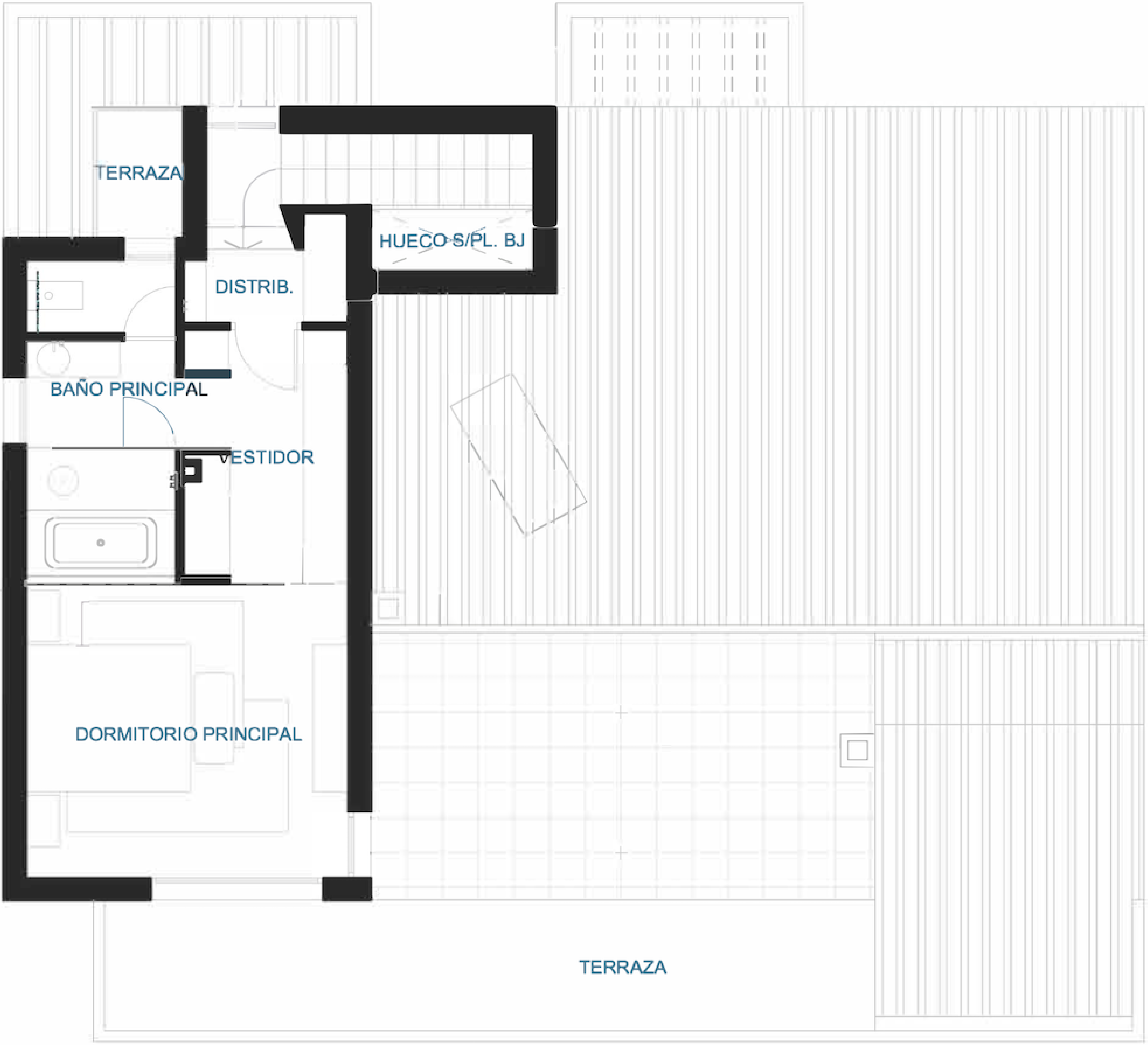
PLANTA PRIMERA
