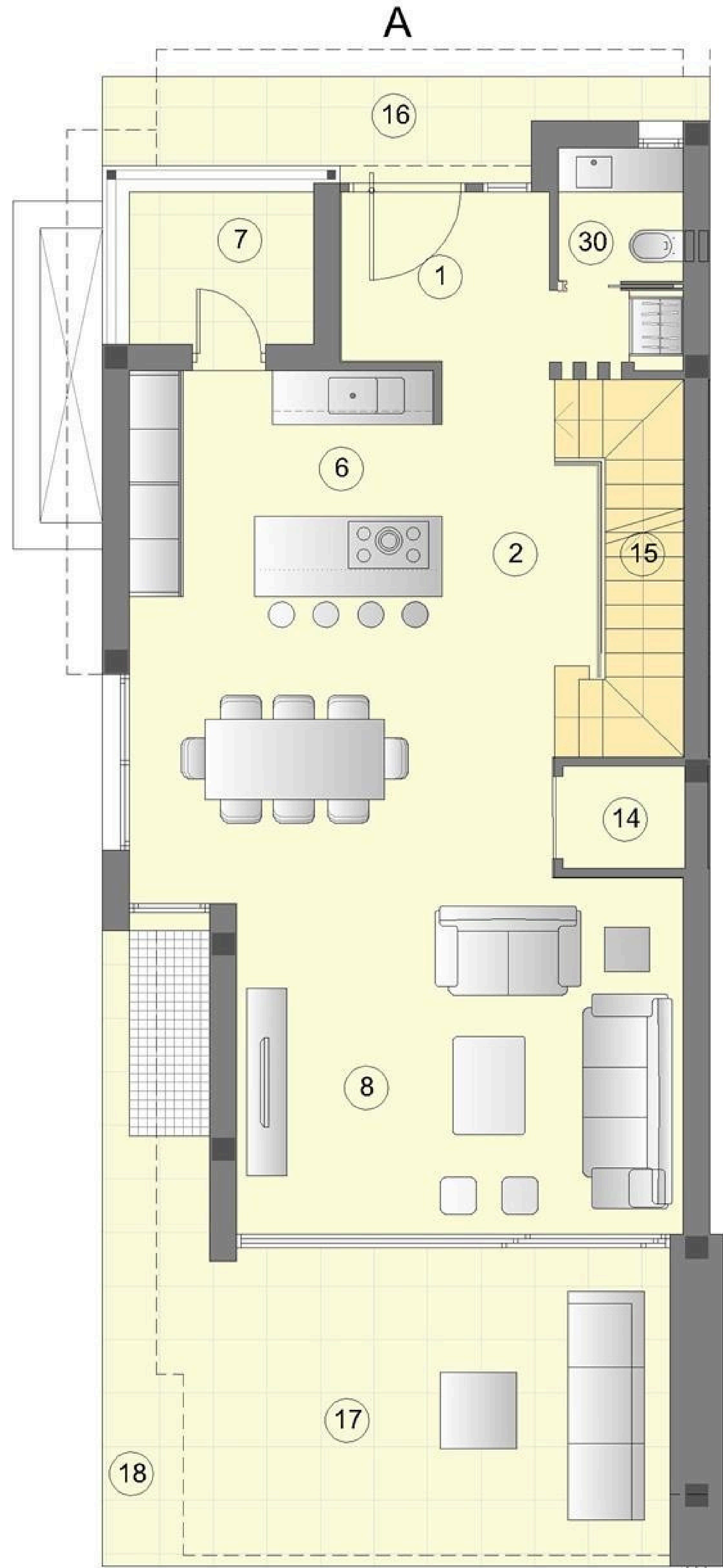
PLANTA BAJA
