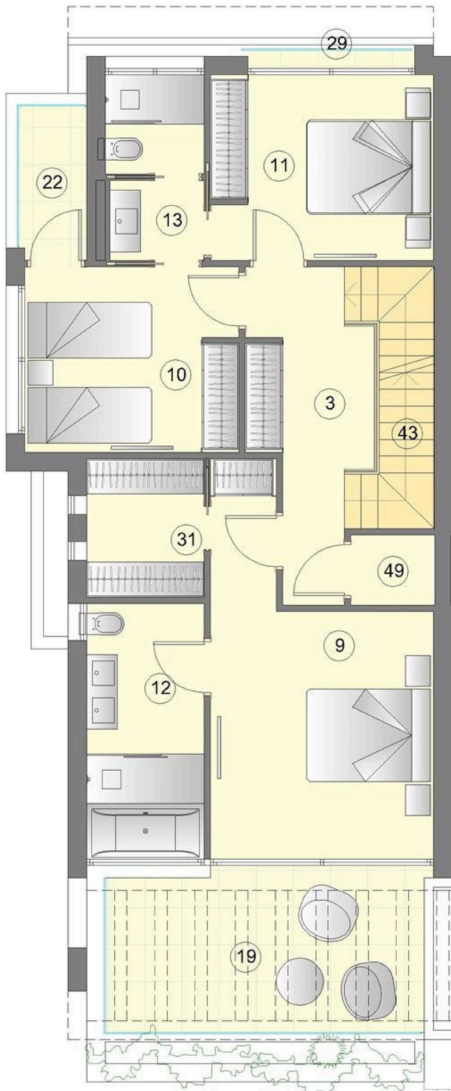
PLANTA PRIMERA
