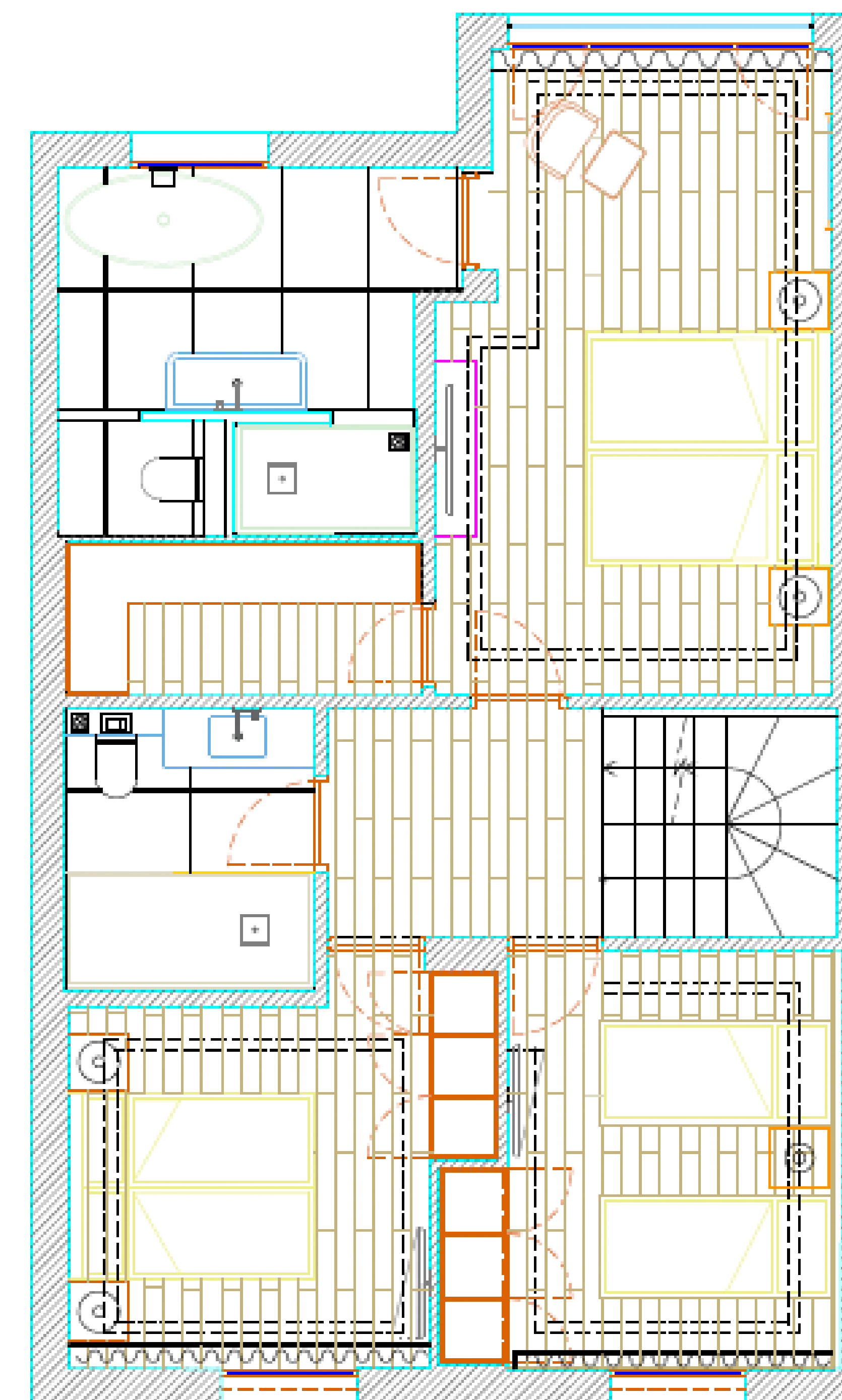
PLANTA PRIMERA. DISTRIBUCION
