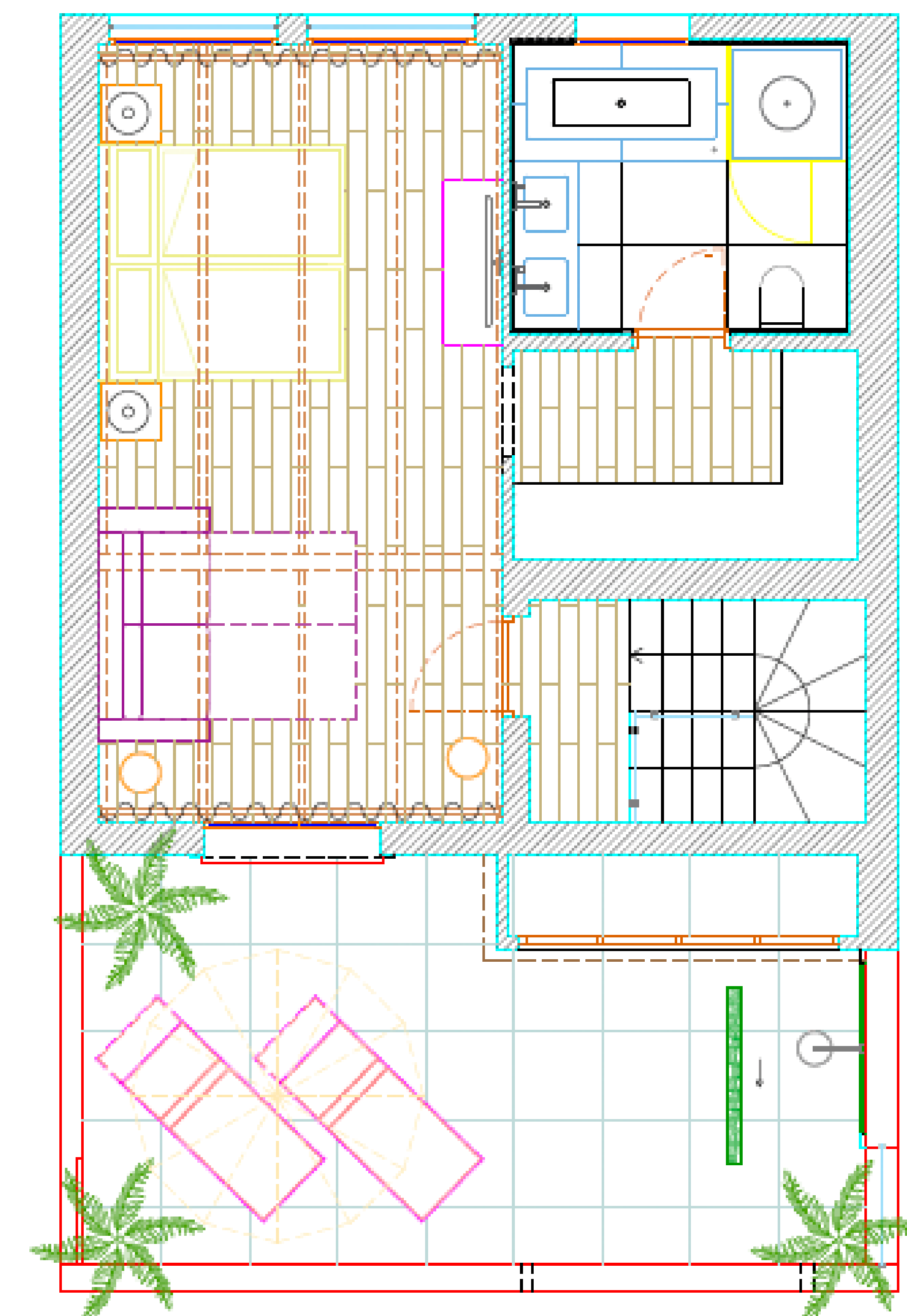
PLANTA SEGUNDA. DISTRIBUCION
