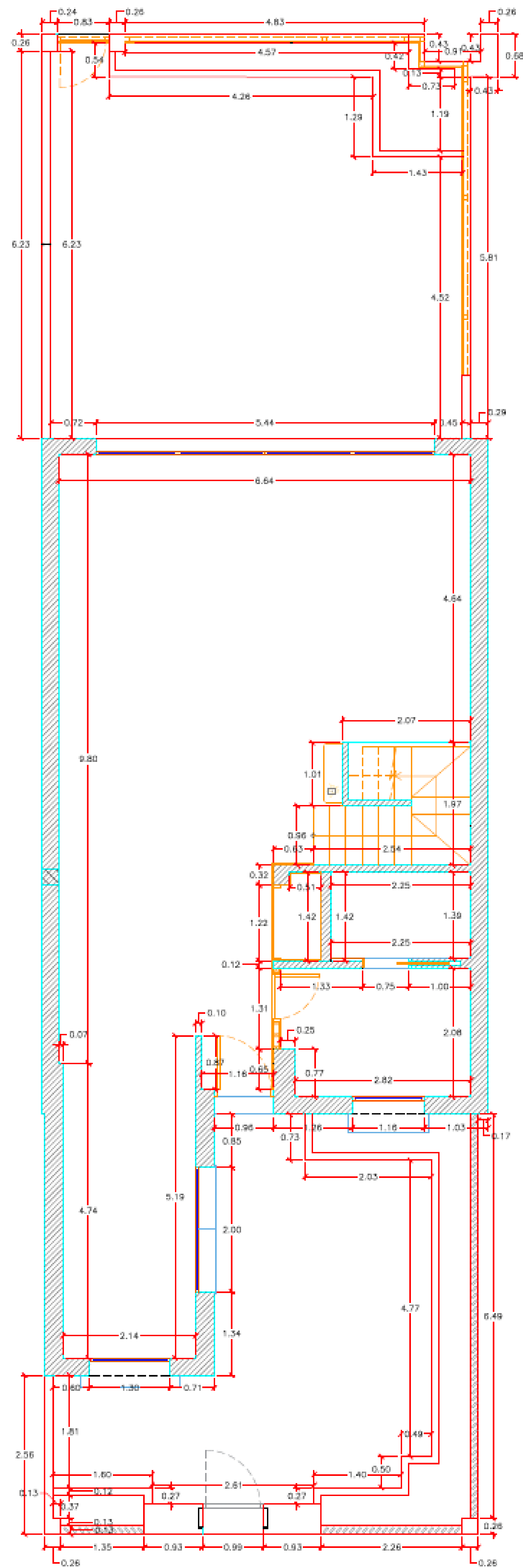
PLANTA PRIMERA. COTAS
