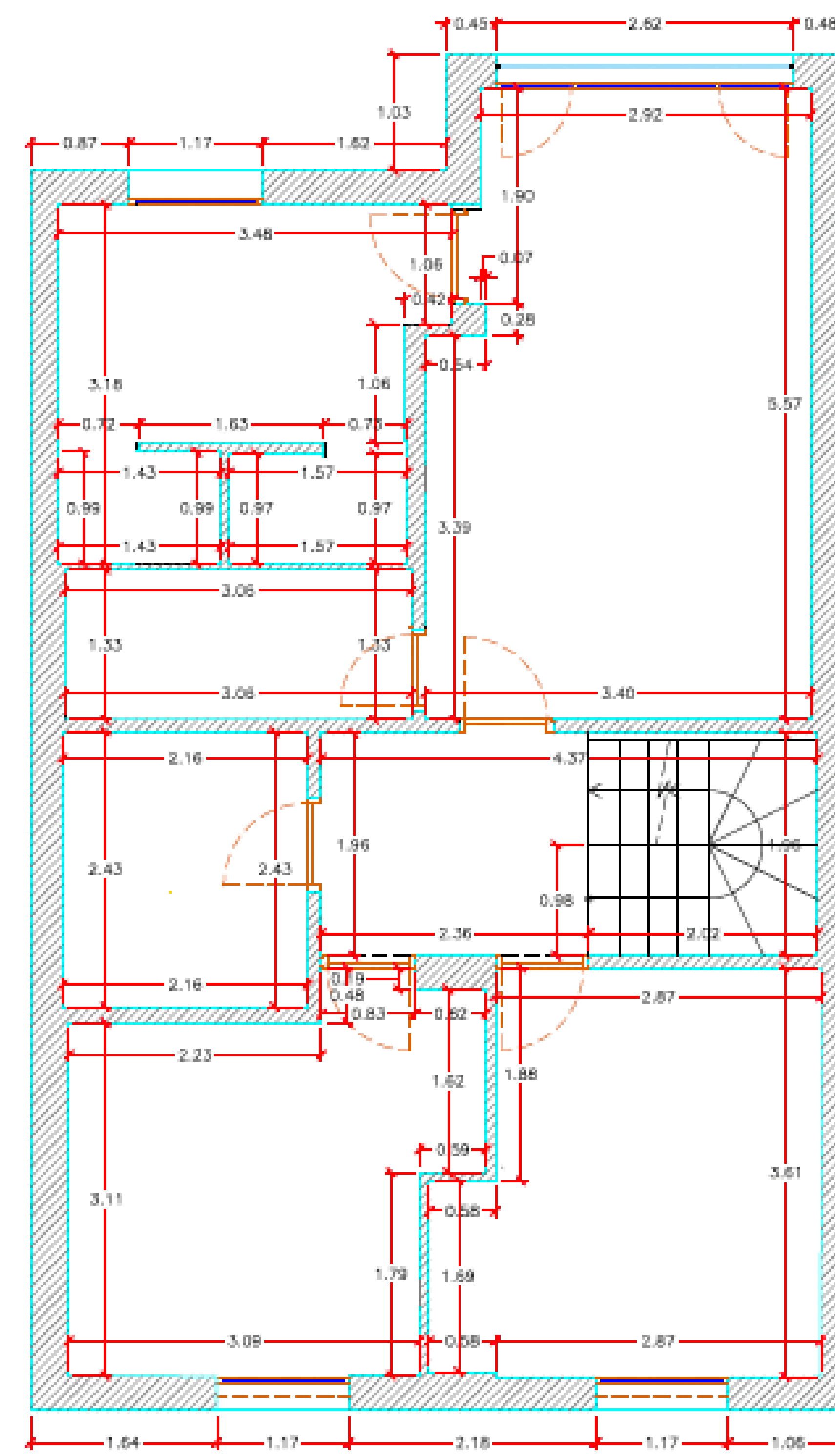
PLANTA SEGUNDA. COTAS
