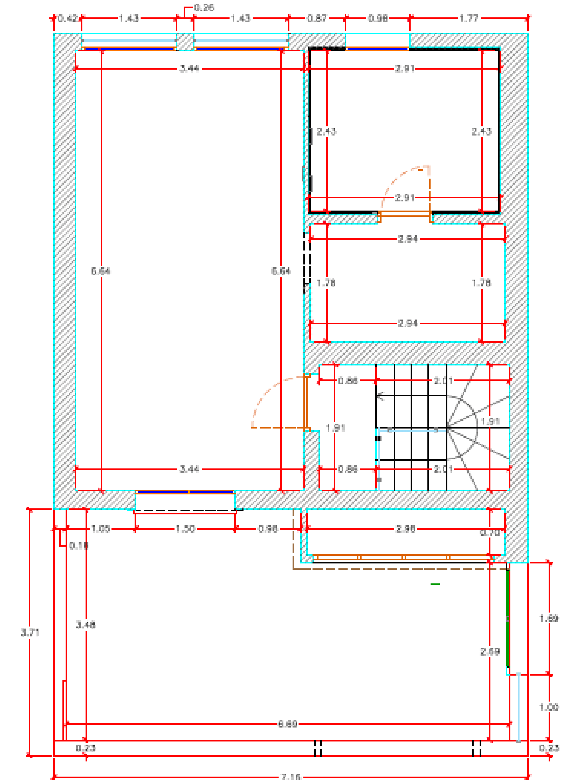
PLANTA TERCERA. COTAS
