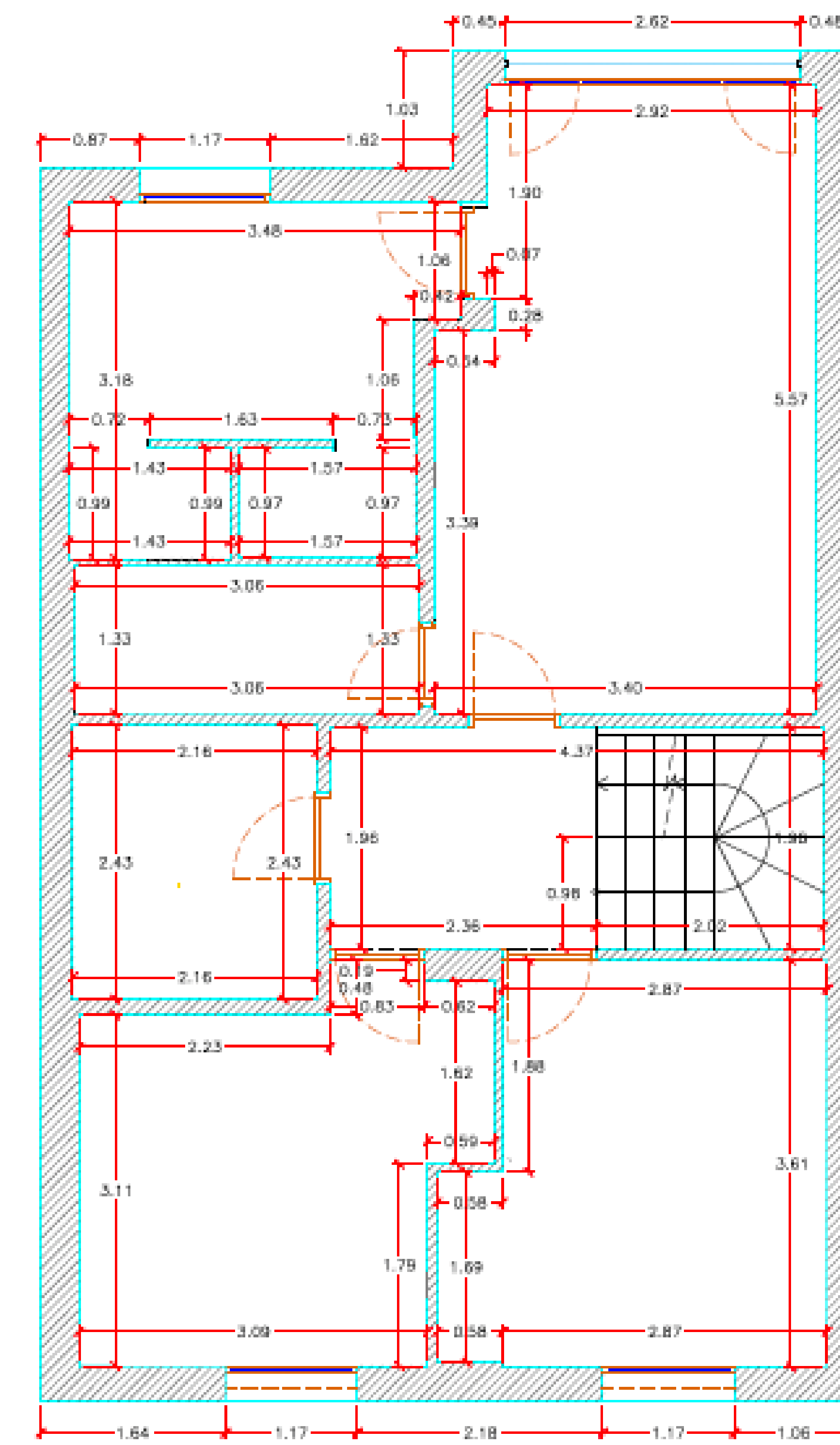
PLANTA PRIMERA. COTAS
