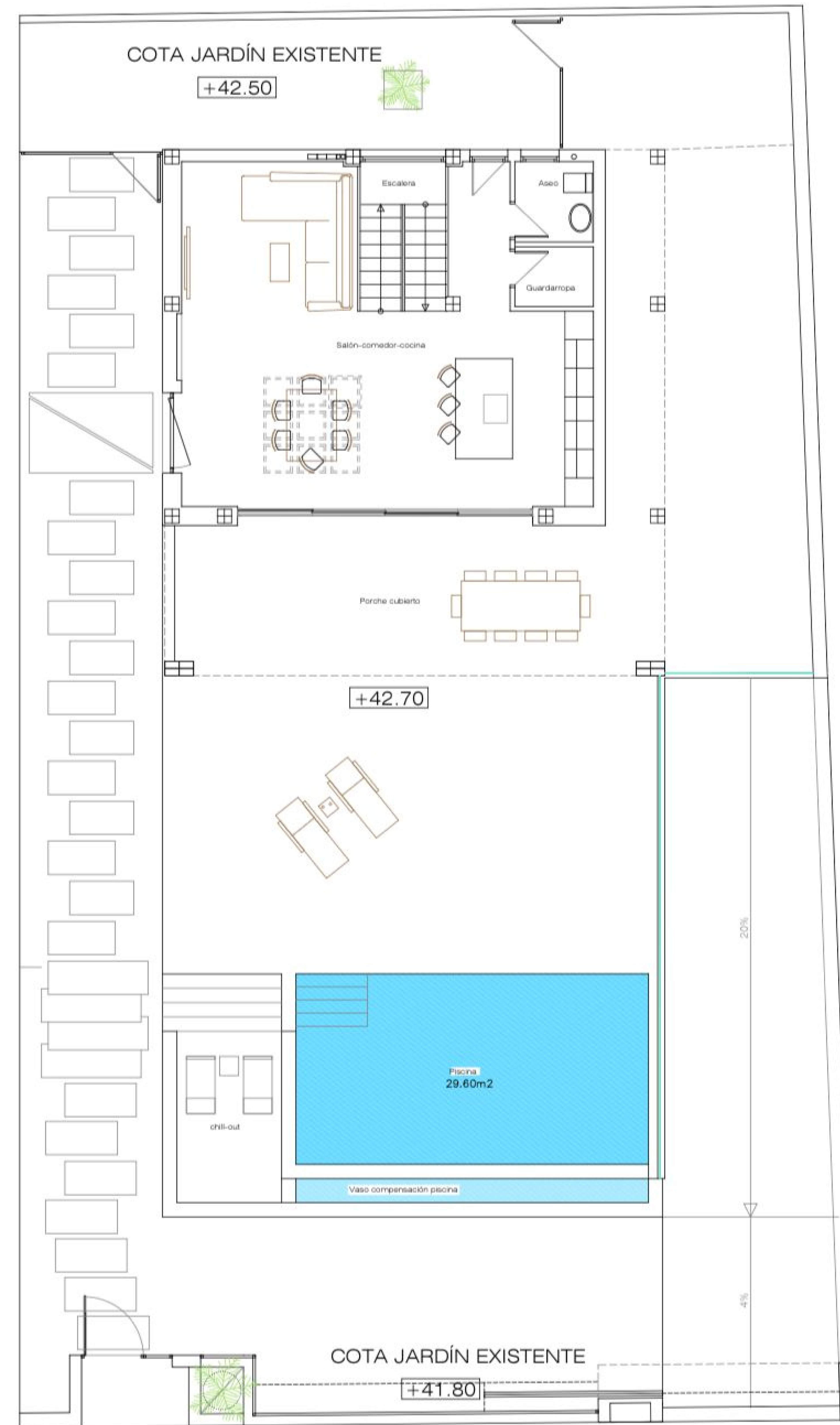
PLANTA BAJA Y DE CONJUNTO
