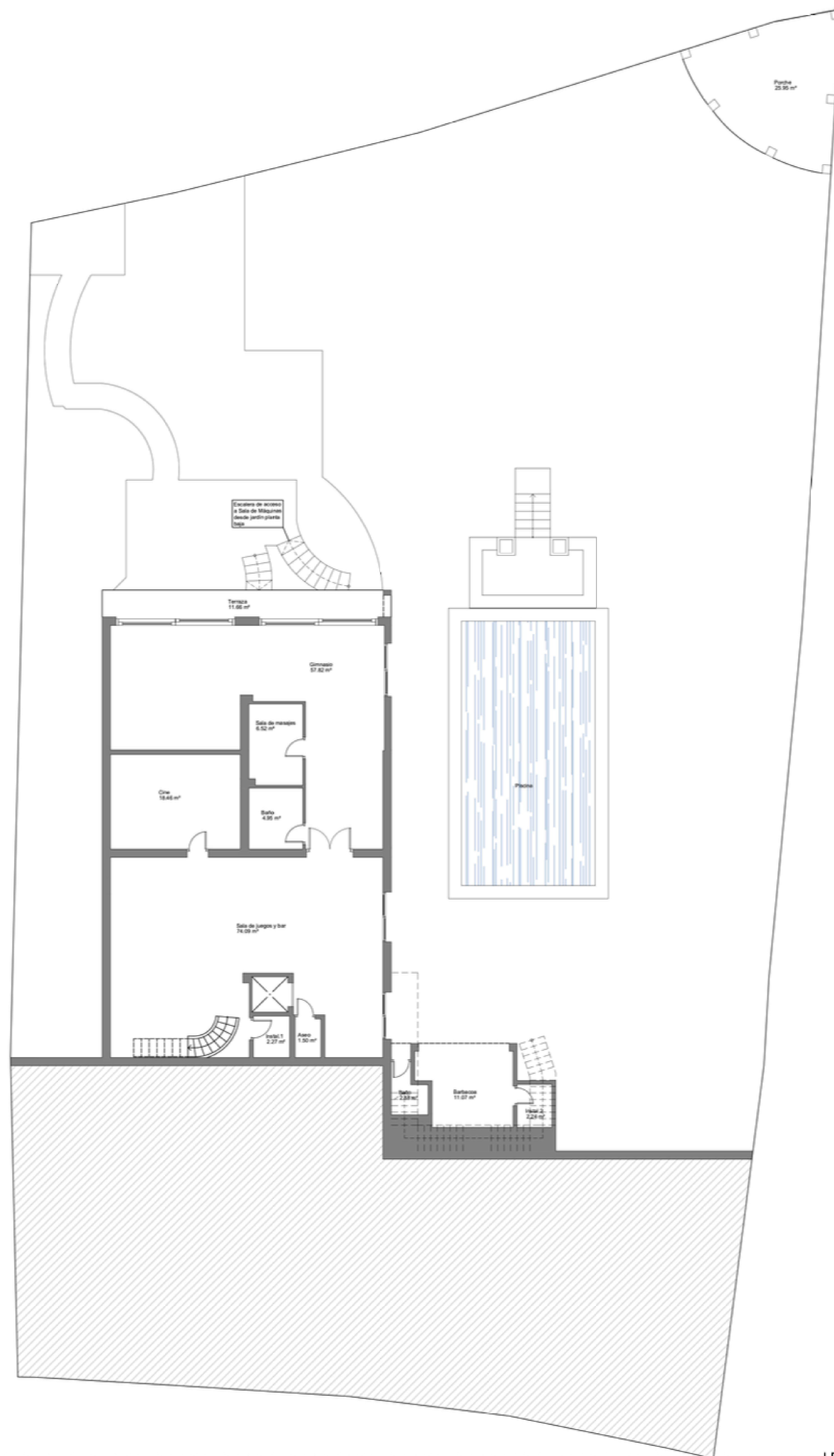
LEVEL - 2 PLANTA -2
