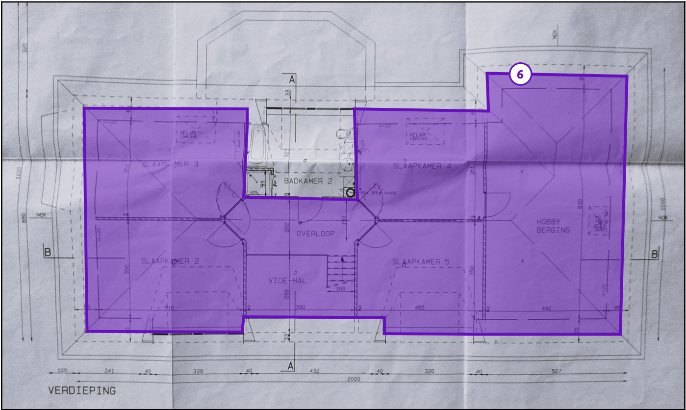
Legende van plan 1.8: vloerplan v+1
