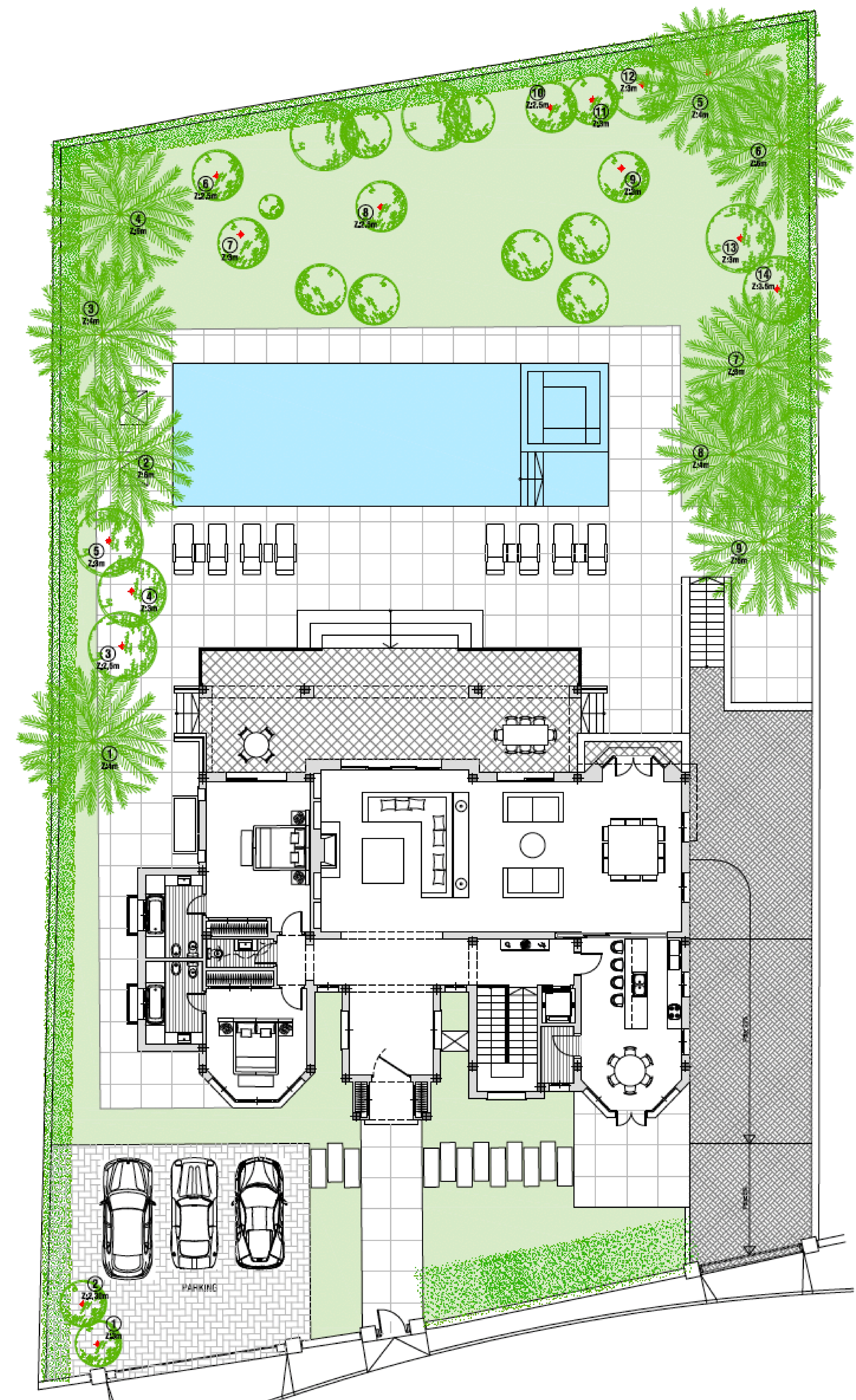
EMPLAZAMIENTO. PLANTA BAJA
