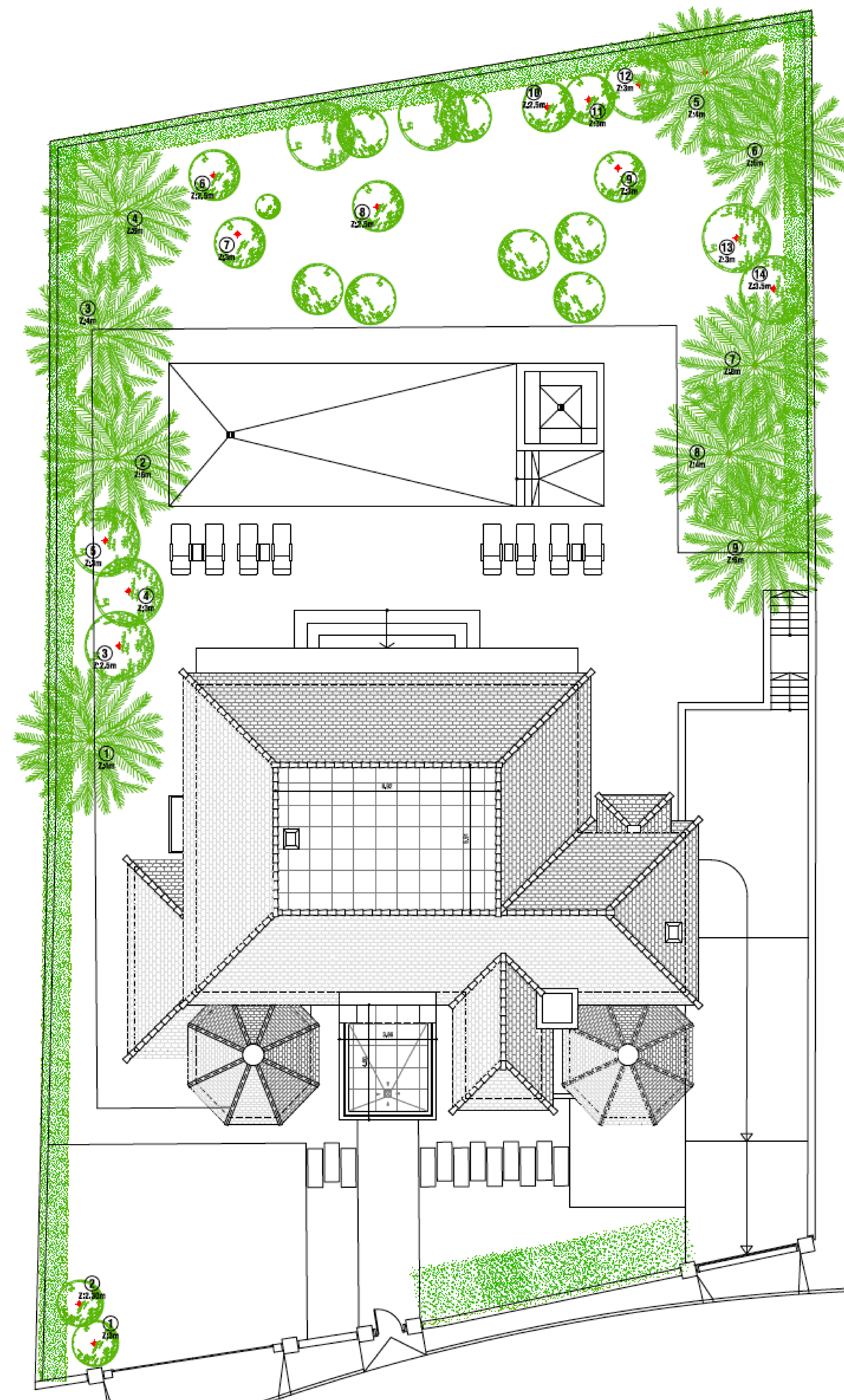
EMPLAZAMIENTO. PLANTA CUBIERTA
