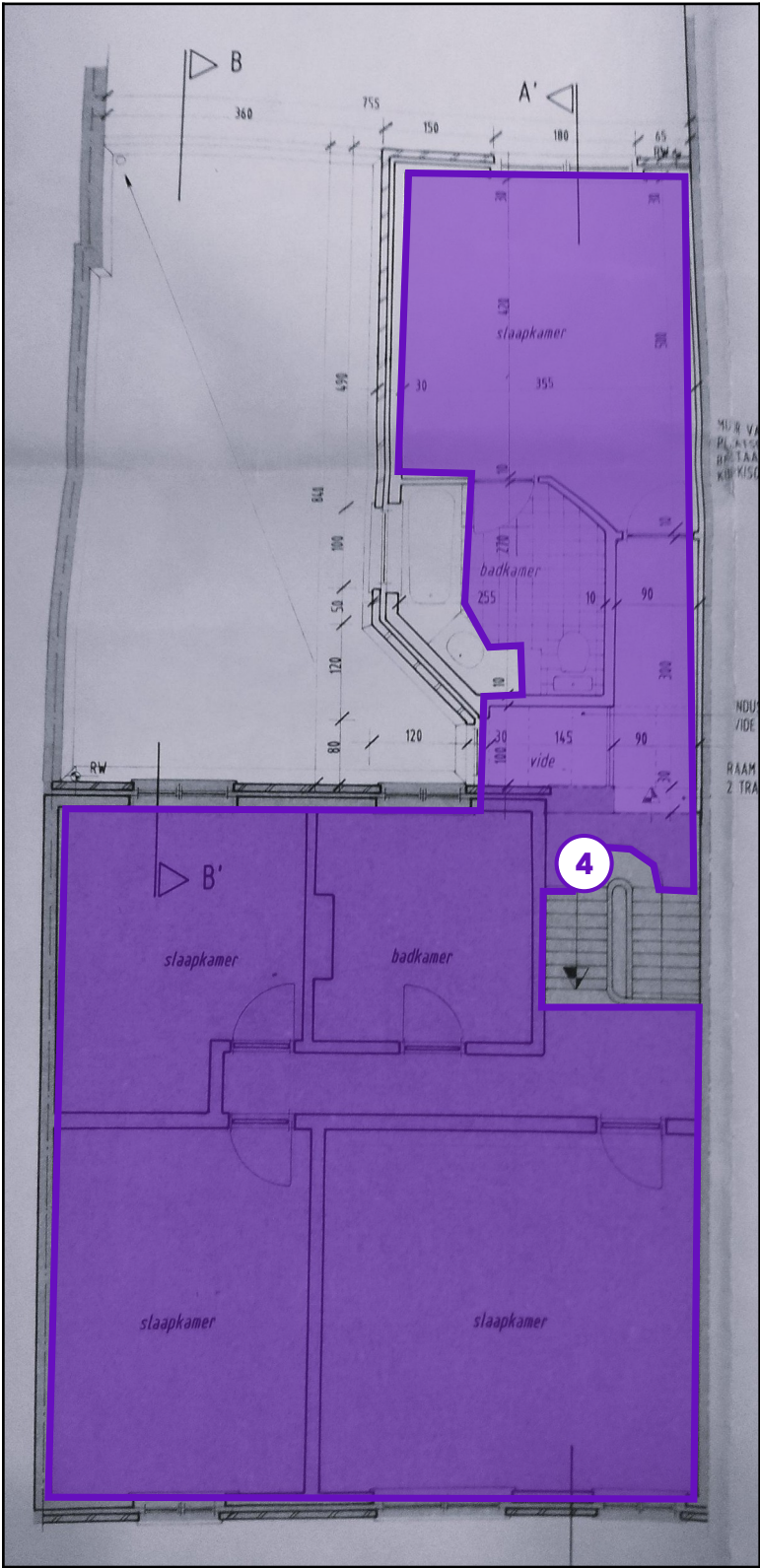
Legende van plan 1.6: VLOERPLAN V+1
