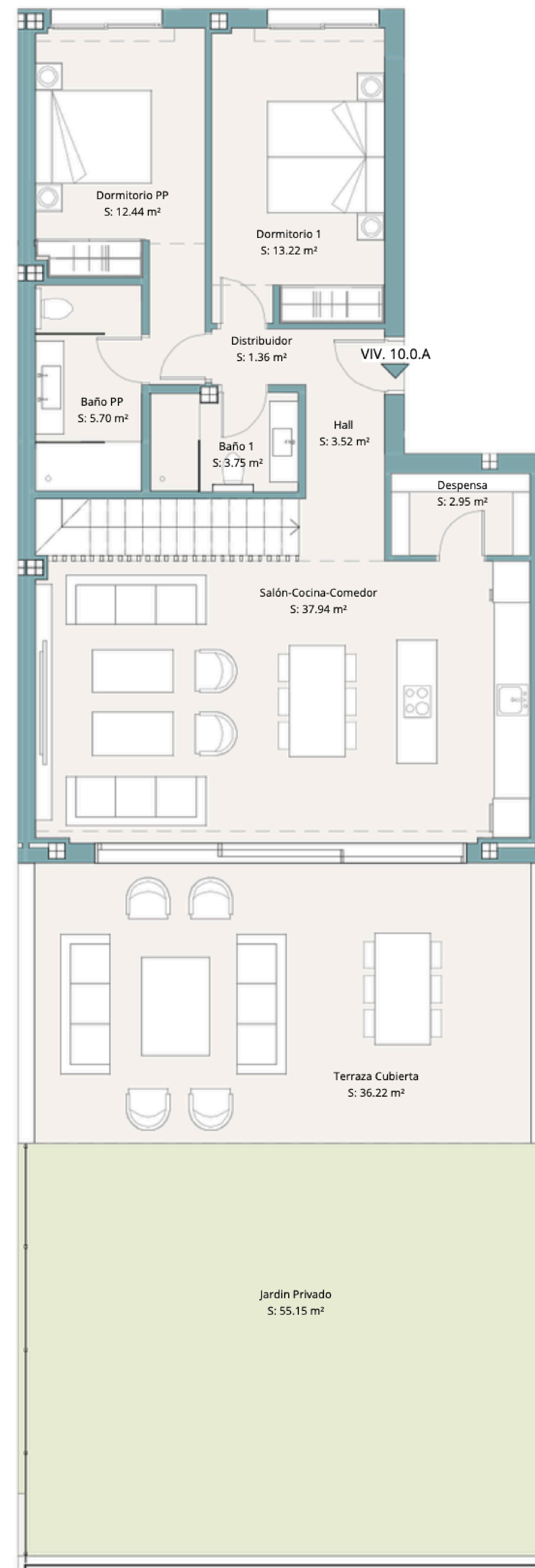
PLANTA BAJA
