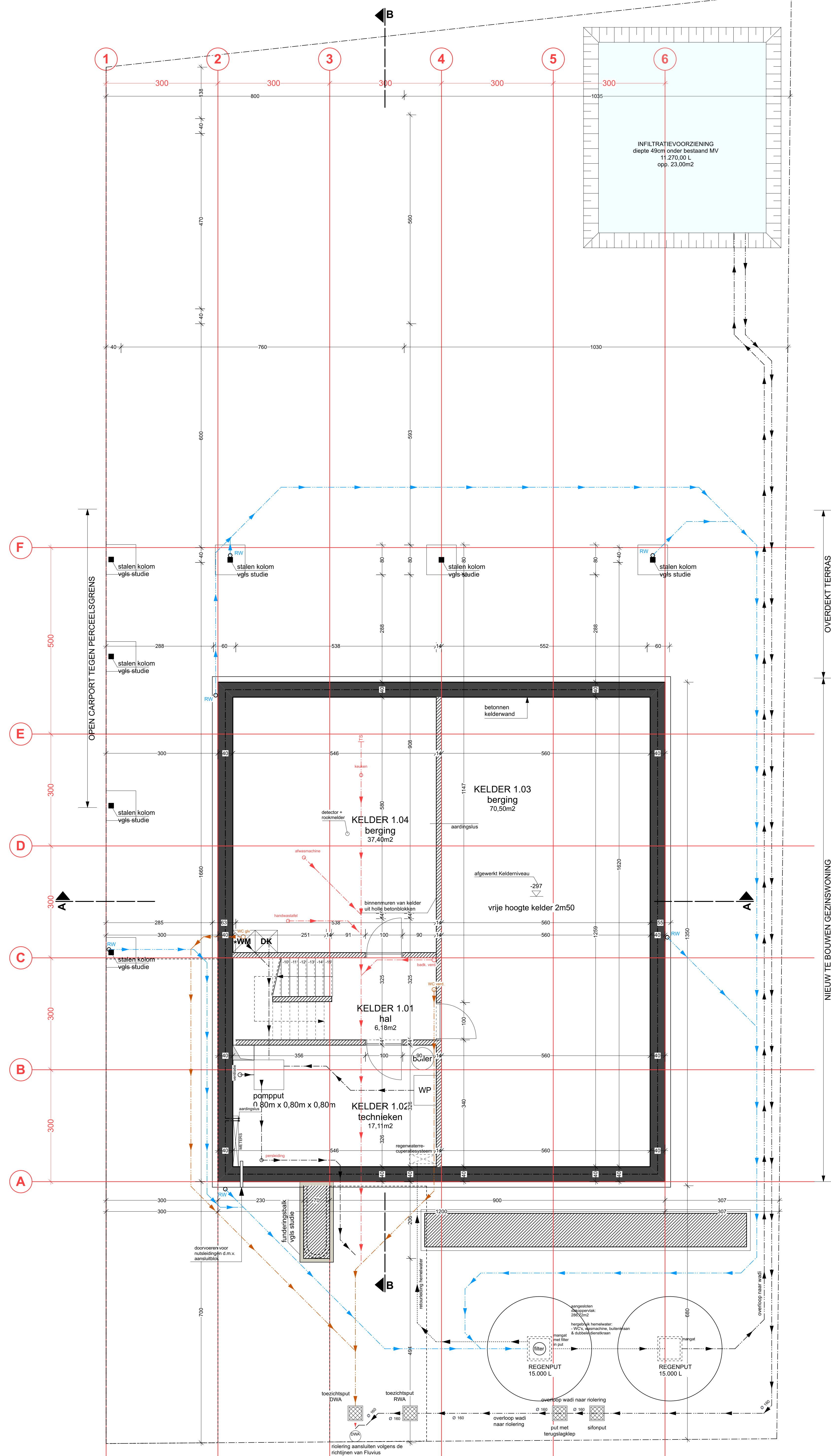
KELDER- EN RIOLERINGSPLAN
